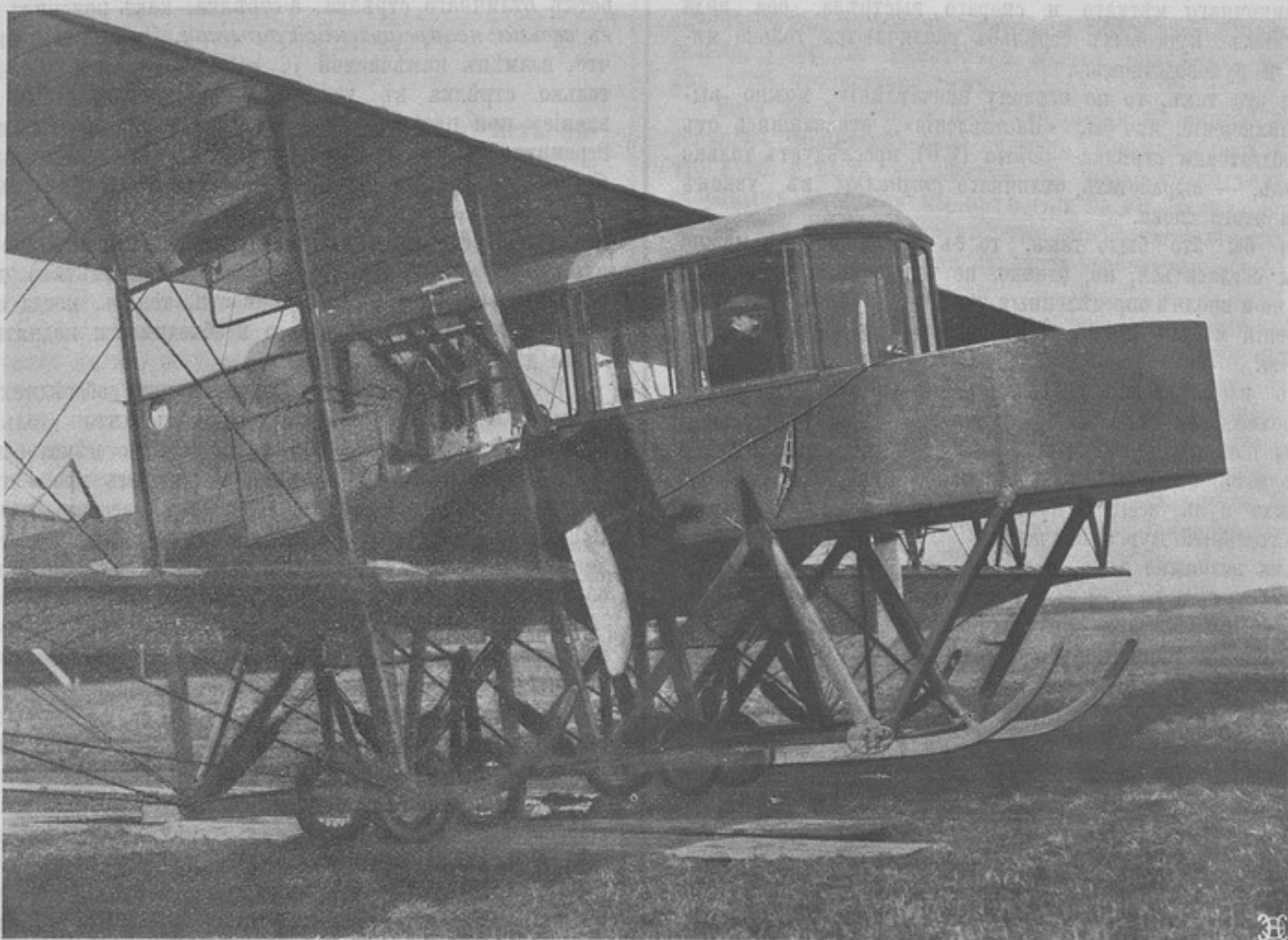
Изъ поѣздки военного министра, генераль-адъютанта Сухомлинова, въ апрѣлѣ с. г. въ Ригу. Осмотръ аэроплановъ.
