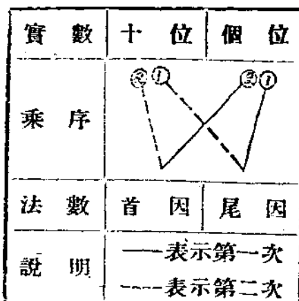
法數兩位乘法乘序圖
