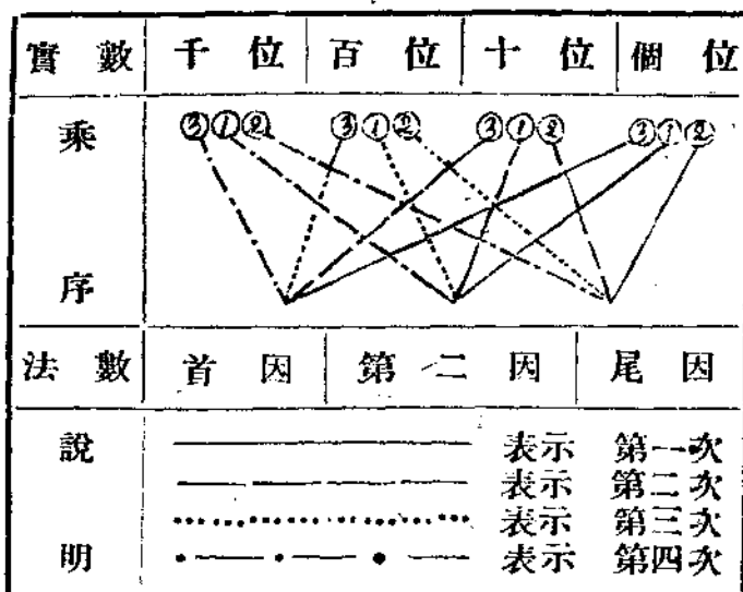
多位乘法乘序圖
