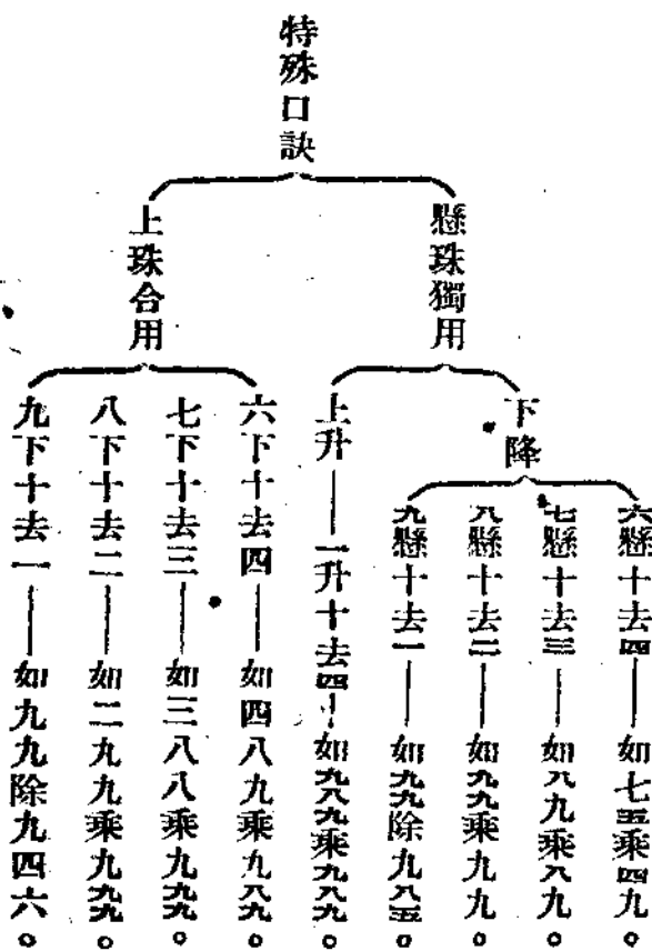
乘除法特殊口訣表(表十一)
