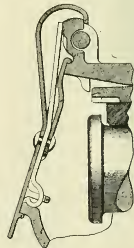
JOURNAL BOX LID.
