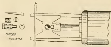
PISTON ROD PULLER.
