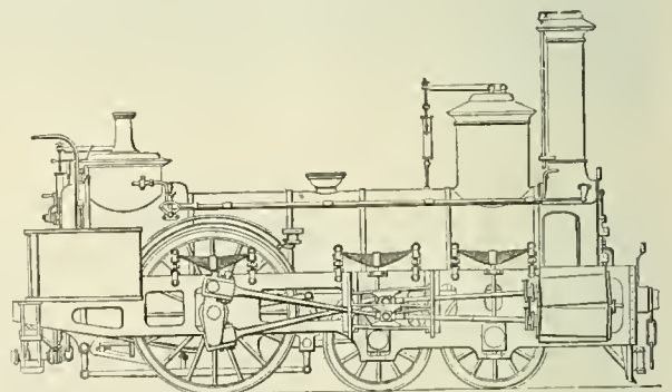
FIG. 13. "DUPLIX," AUSTRIA, 1861.
