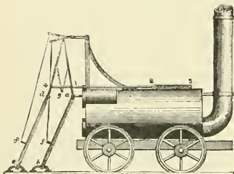
FIG. 1. BRUNTON'S TRAVELLER, 1813.
