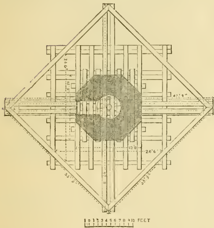
Fig. 3.—Plan.
