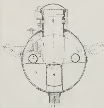
Fig. 3.—Sección transversal del submarino. — 1. Aparato para abrir y cerrar la capota. — 2. Capota de descenso. — 3. Caja de agua lateral. — 4. Caja de agua central. — 5. Depósitos de aire comprimido. — 6. Remos. — 7. Juntas esféricas. — 8. Plomada de seguridad.
