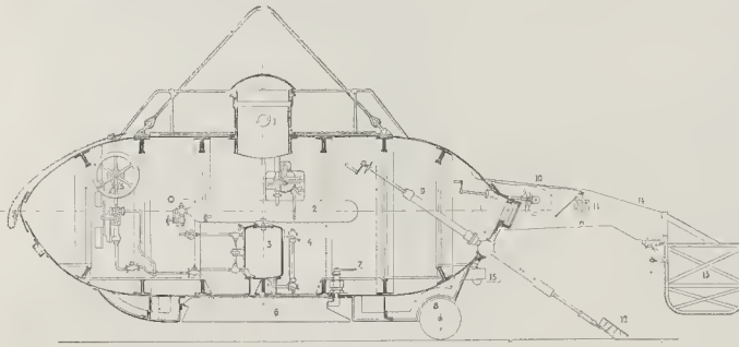
Fig. 2.—Sección longitudinal del submarino. — 1. Capota de descenso. — 2. Depósito de aire comprimido. — 3. Caja de agua central. — 4. Caja de agua lateral. — 5. Bomba. — 6. Plomada de seguridad. — 7. Válvula de la plomada de seguridad. — 8. Rueda. — 9. Brazo móvil. — 10. Cabria de maniobra de la plomada de anclaje. — 11. Lámparas eléctricas. — 12. Pinza para coger las esponjas. — 13. Cesta. — 14. Brazo. — 15. Plomada de anclaje.
