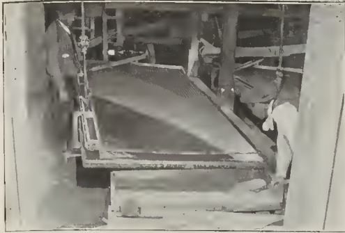
Taller de lavado y separación mecánica del mineral fino
