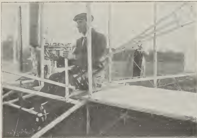
Mr. Wilbur Wright haciendo funcionar las palancas de dirección de su aeroplano (De fotografía de M. Branger.)
