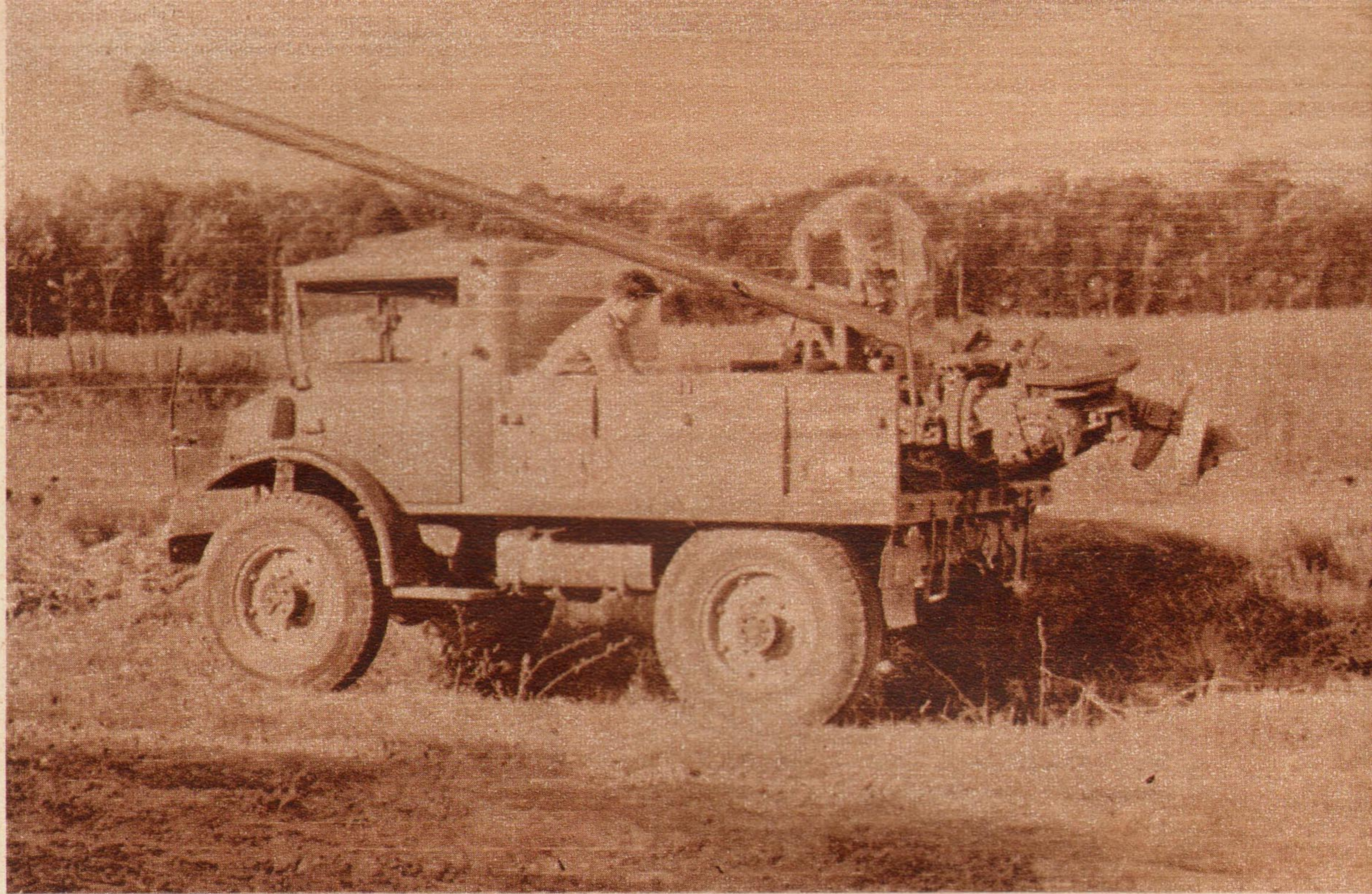
Llegan a 53 las Brigadas Móviles con que cuenta Teléfonos del Estado. Cada una de ellas está compuesta por doce hombres, perfectamente equipados con herramientas de calidad y elementos mecánicos de auxilio, como camiones perforadores de hoyos y colocadores de postes.
