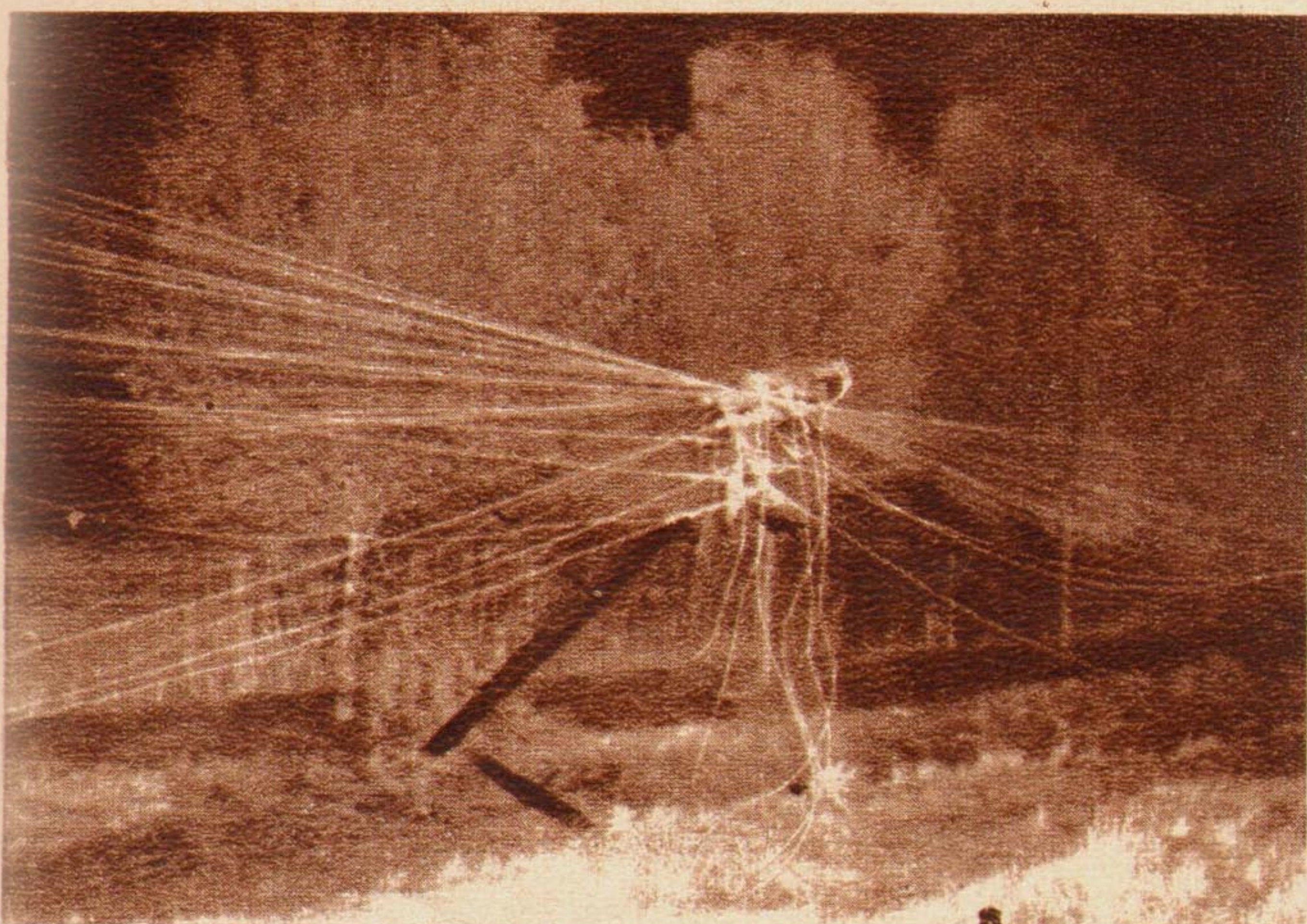
La foto muestra el estado en que quedó uno de los postes de la línea Capital Federal - Mar del Plata, a la altura de Glew, después de la tormenta. Las Brigadas Móviles repararon el daño en sólo cuatro horas.
