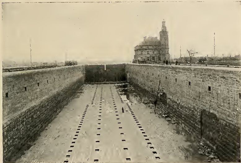
AN EMPTY LOCK—SAULT STE. MARIE CANAL.
