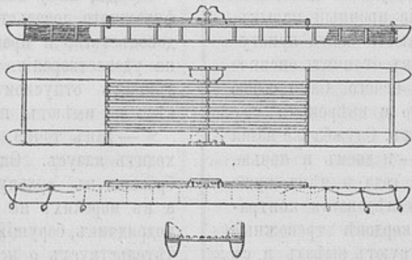
(Къ ст. «Спасательные плоты».)
