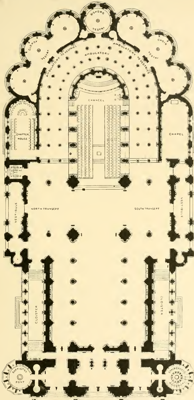
GROUND-PLAN.
