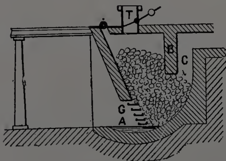
Fig. 2. — Gazogène à barrage.
