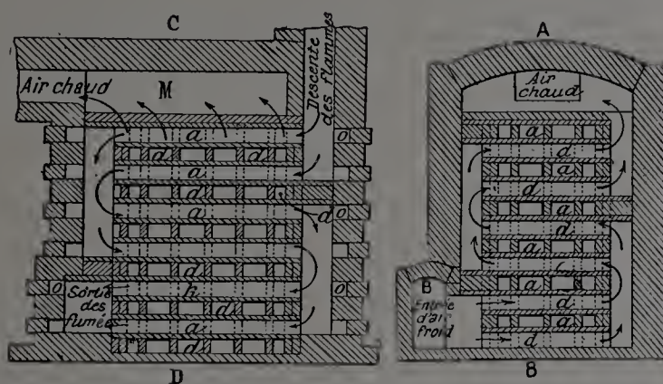
Fig. 15. — Coupe suivant P P
