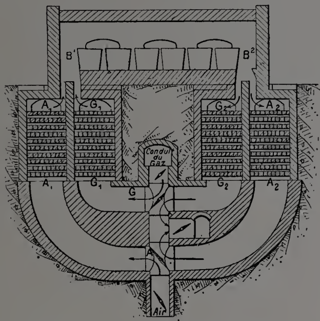
Fig. 18. — Ancien four Siemens.
