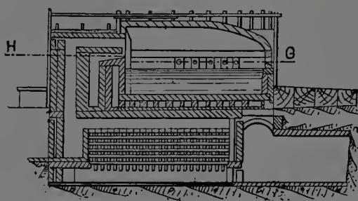
Fig. 19. — Coupe suivant A B
