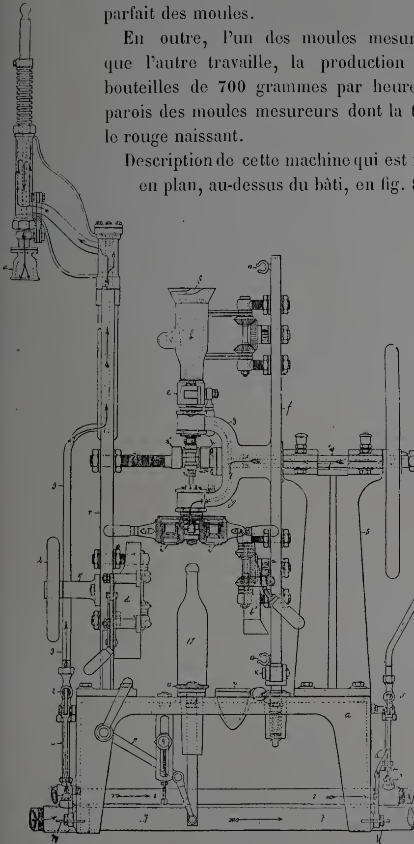
Fig 86. — Machine à double moule ébaucheur. Vue de face au moment où la bouteille est terminée.
