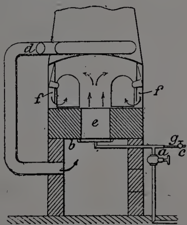
Fig. 21. — Four à gaz naturel de la glacierie d'O'Hara.
