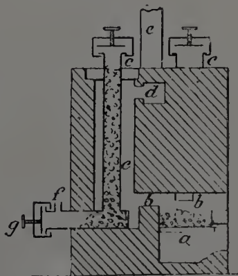
Fig. 7. — Gazogène Riché.
