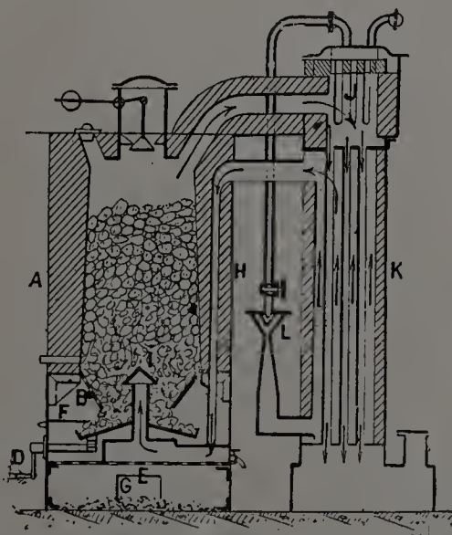
Fig. 4. — Gazogènes Taylor (Fichet et Heurtey)
