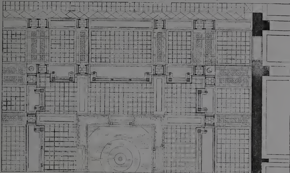
Fig. 138 bis. — Planchers en fer et en verre du premier étage et du rez-de-chaussée.
