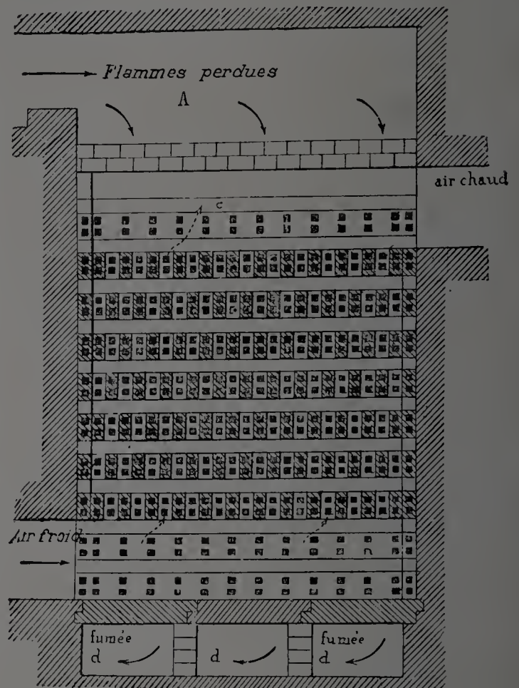
Fig. 14. — Coupe suivant C D.
