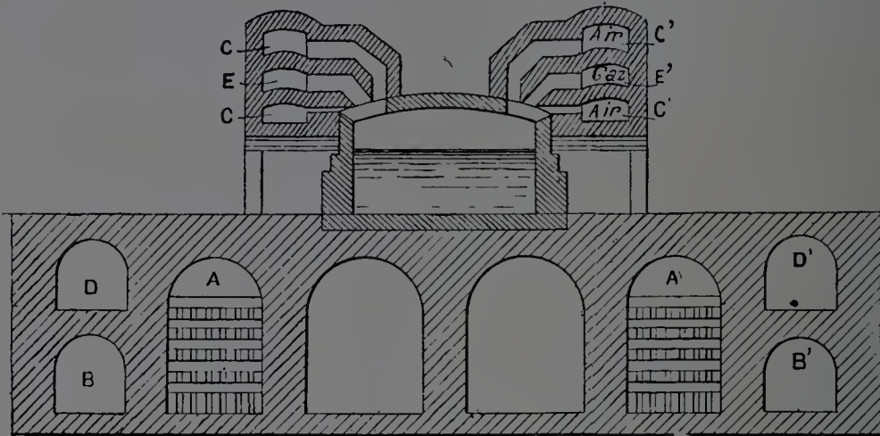
Fig. 17. — Four Gobbe (Coupe transversale).
