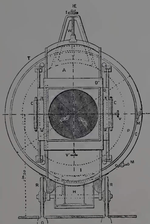
Fig. 79. — Vue de face de l'oculaire
