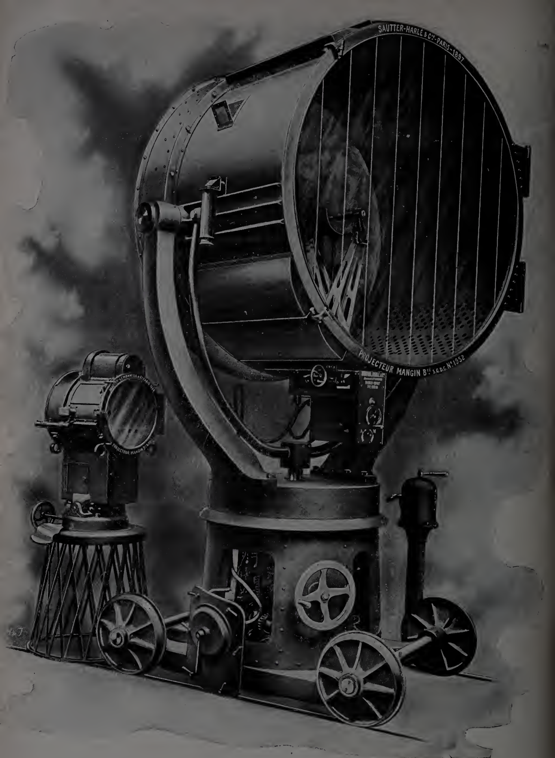
Fig. 57. — Projecteur Mangin.
