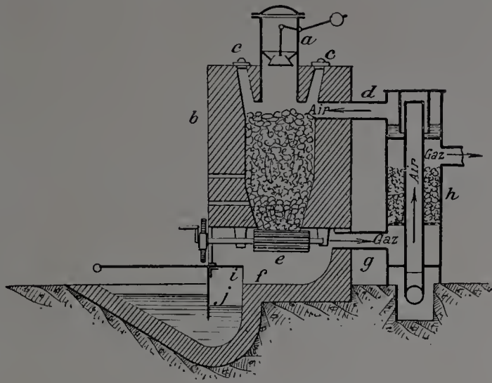
Fig. 5. — Gazogène Faugé.
