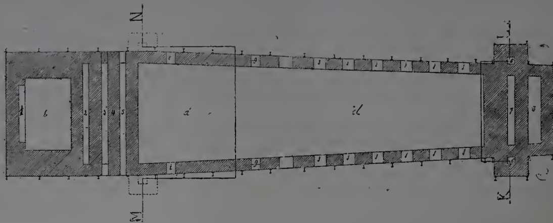
Fig. 95. — Coupe horizontale.
