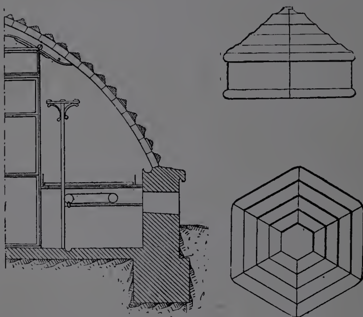
Fig. 33. — Briques creuses en verre (système Falconnot).
