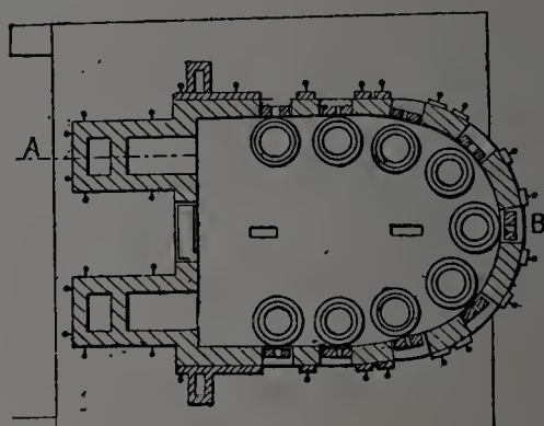
Fig. 20. — Coupe horizontale suivant H G
