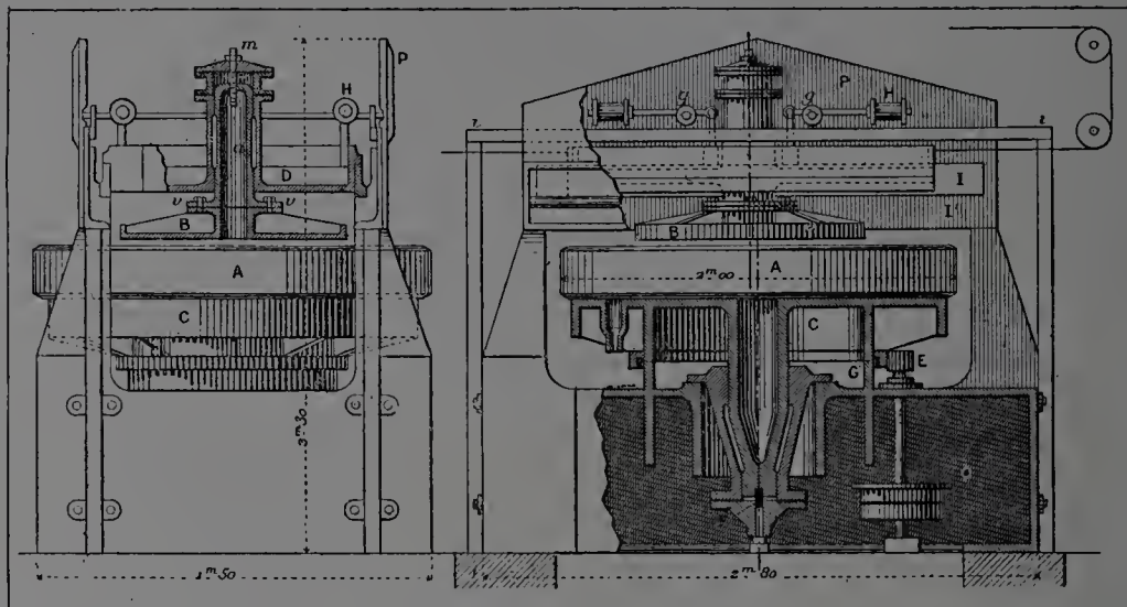
Fig. 80. — Machine à travailler mécaniquement les surfaces optiques.
