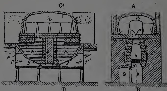
Four Boétius. — Fig. 8. — Coupe selon A B. — Fig. 9. — Coupe selon C D.
