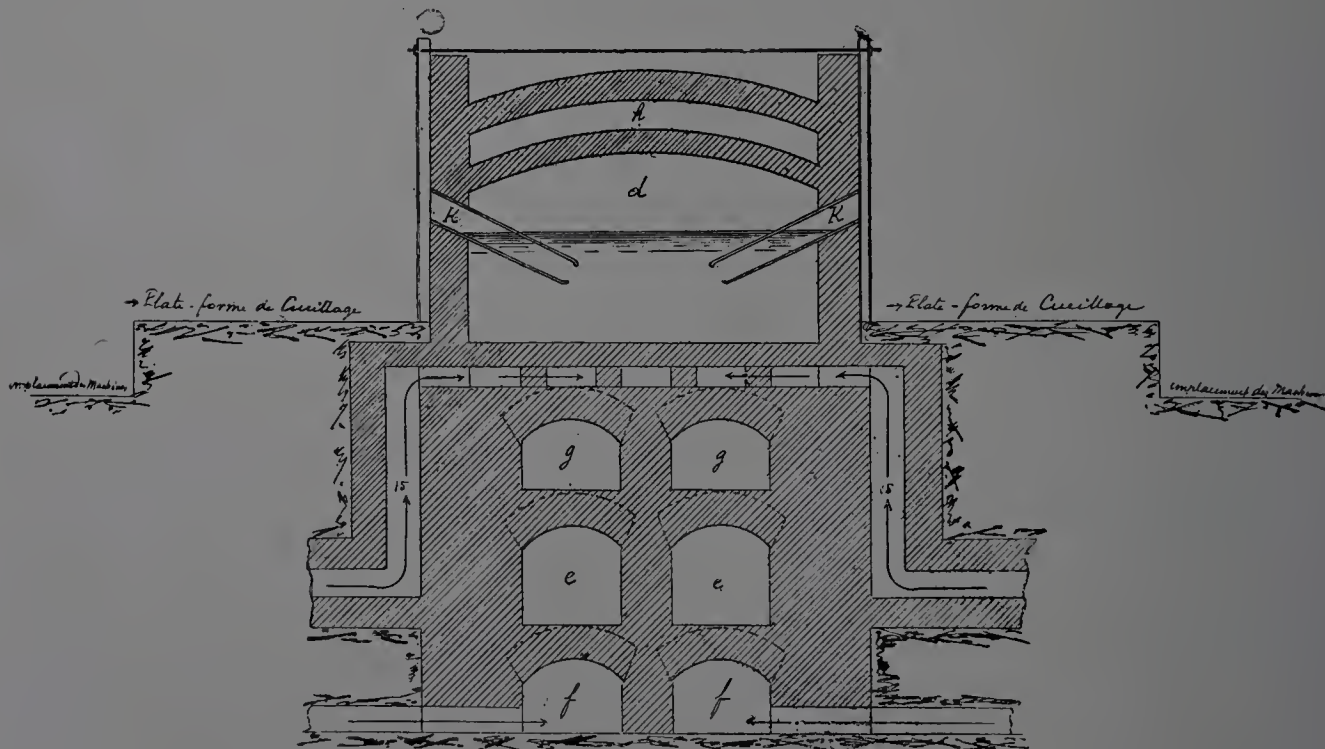
Fig. 96. — Coupo transversale par los ouvreaux de cueillage laissant voir en même temps les conduits 15 dans lesquels l'air s'élève pour pénétrer derrière l'autel sous la sole du bassin.
