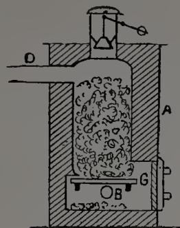
Fig. 3. — Gazogène Dowson
