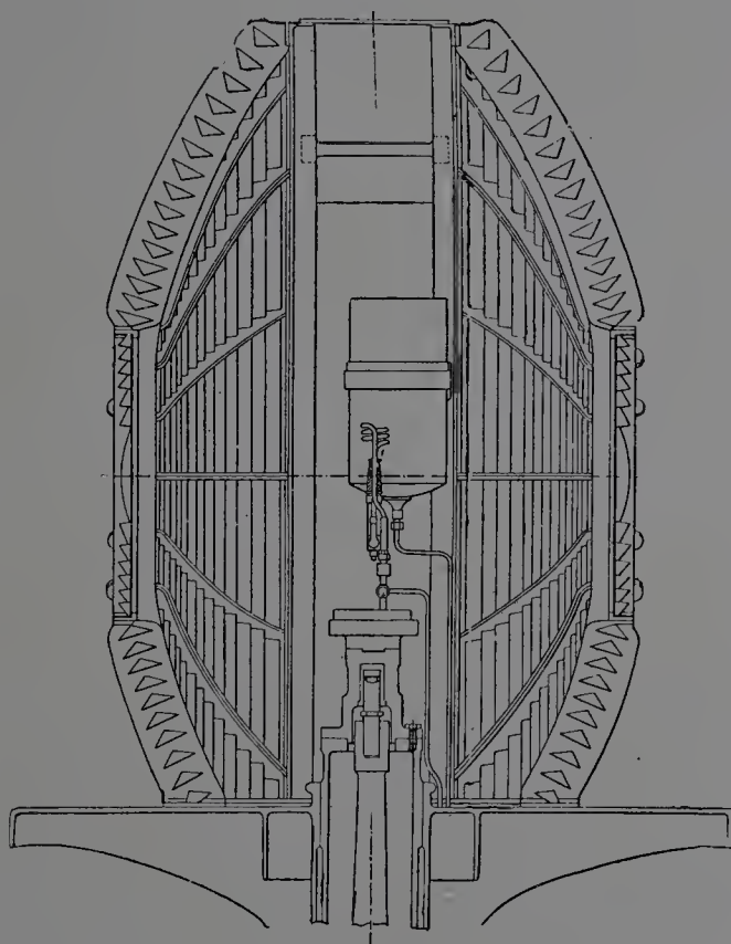
Fig. 55. — Feu éclair à deux éclats (coupe longitudinale.)
