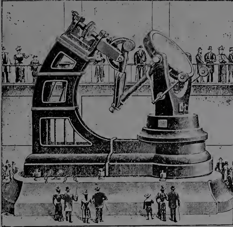
Fig. 75. — Le sidérostat [de la grande lunette.
