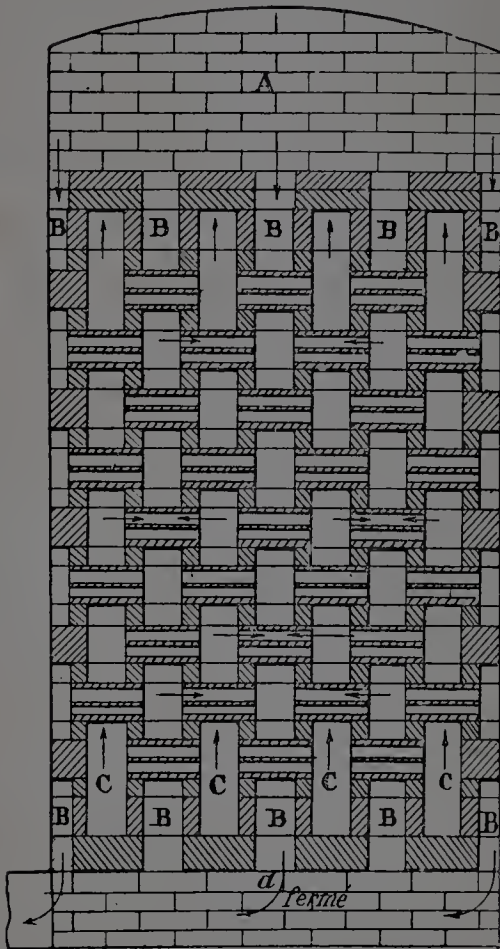
Fig. 13. — Coupe suivant A B.
