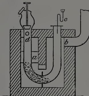
Fig. 6. — Gazogène Guénot.
