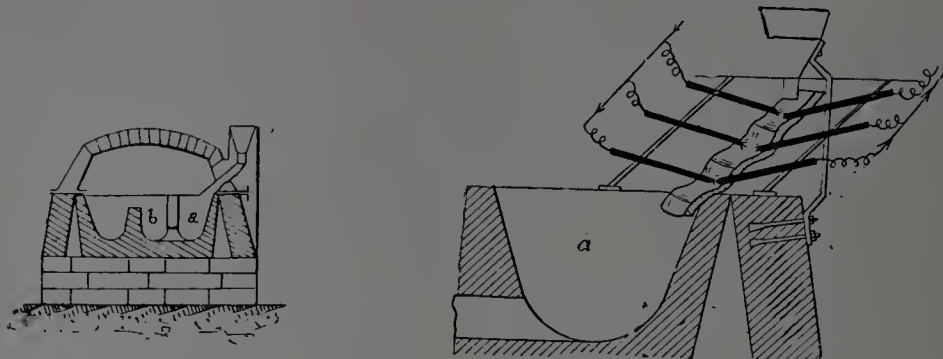
Fig. 24. — Four primitif. Coupe verticale. — Détail du chenal de fusion.
