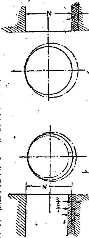
片側公差
