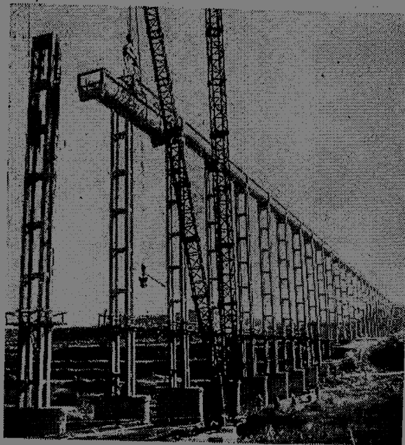
石门县大搞水利工程 配套，充分发挥现有水利工程 效益。这是思于潭渡槽正在施 工。 周克勤摄
