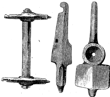
Копыль съ трехъ сторонъ.
