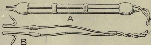
FIG. 24. Hand electrodes.
