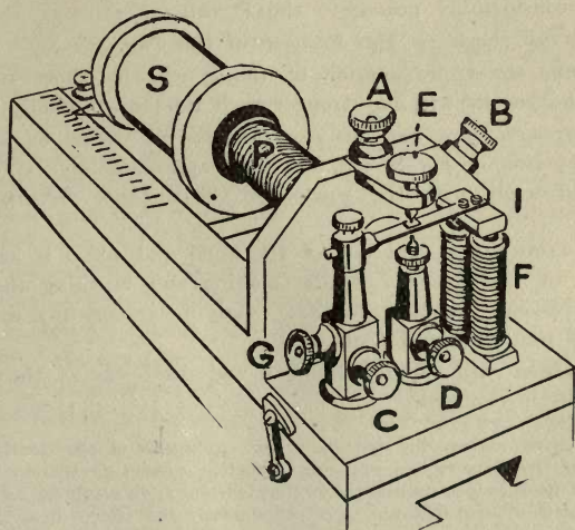
FIG. 26. Inductorium of du Bois Reymond.
