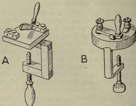
FIG. 21. A Du Bois Reymond, B Simple key.
