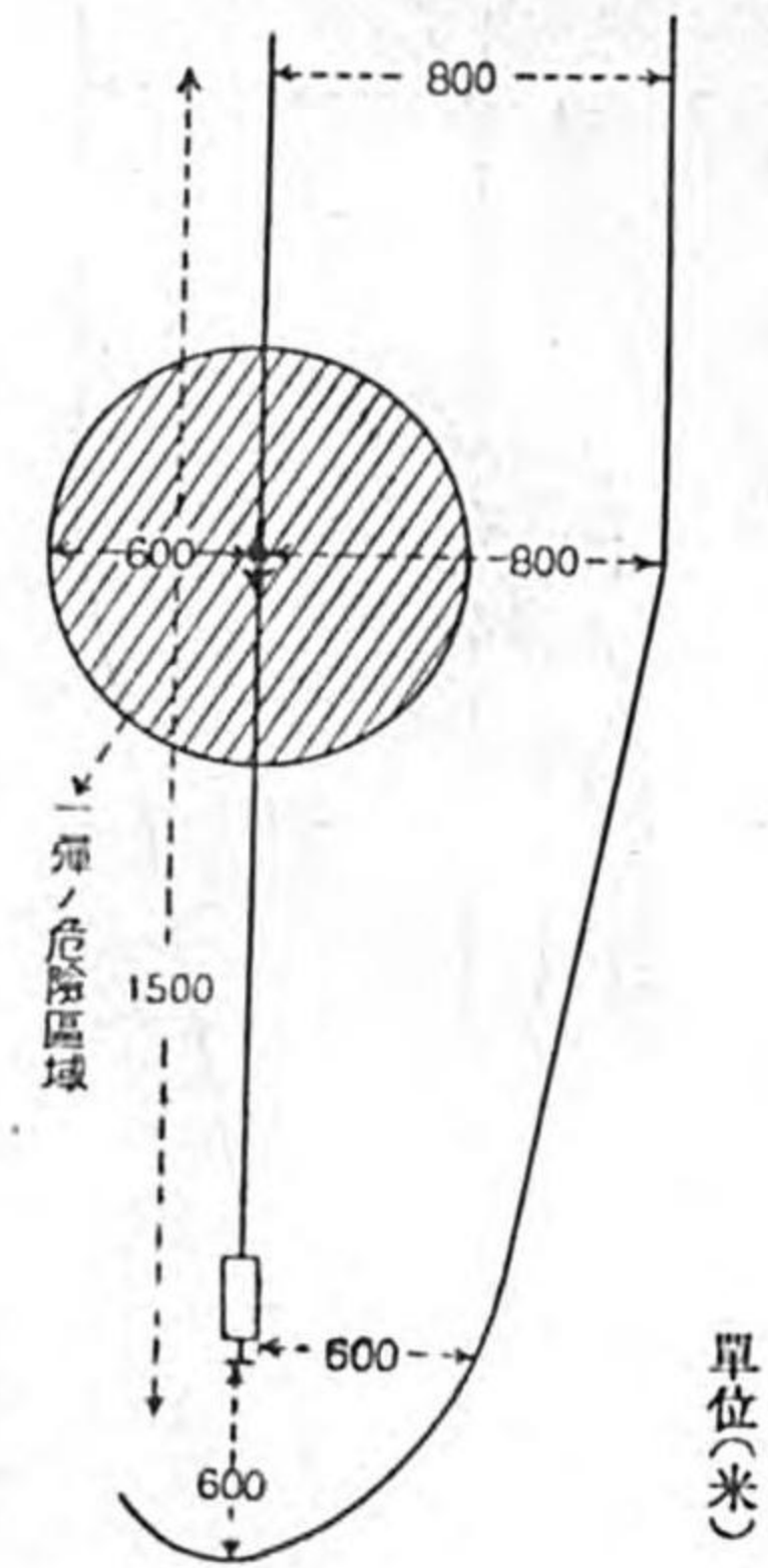
第八圖 榴彈ヲ使用スル場合
