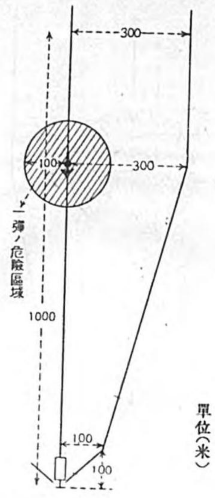
第七圖 代用彈若クハ砂彈ヲ使用スル場合
