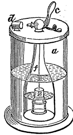
DOBÉREINER'S LAMP.
