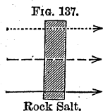
Fig. 137. Rock Salt.
