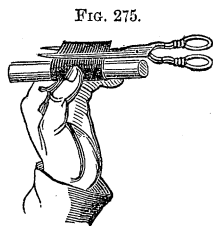
FIG. 275. Cohesion of Caoutchouc.
