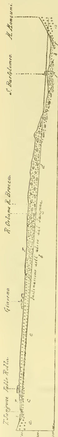
Profilo fra il Sangone, ad ovest di Giaveno e il Moncuni (La pendenza dell'altico del Sangone è proiettata sul piano del profilo). a , roccia in posto; b , Morenico della prima fase glaciale; c , Diluvium superiore; d , Morenico della seconda fase glaciale; e , Morenico della terza fase glaciale; h , torba; i , Alluvium antico; f , Ferretto. Scala: per le altezze 13.300; per le lunghezze 33.300.
