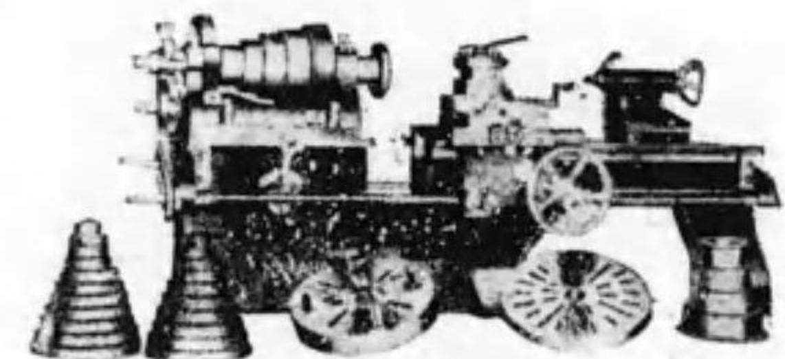
高級八呎旋盤
