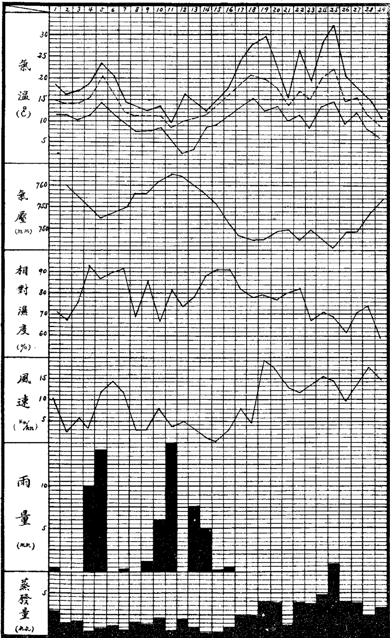
民國二十五年二月份南寧各項氣象要素逐日變遷圖
