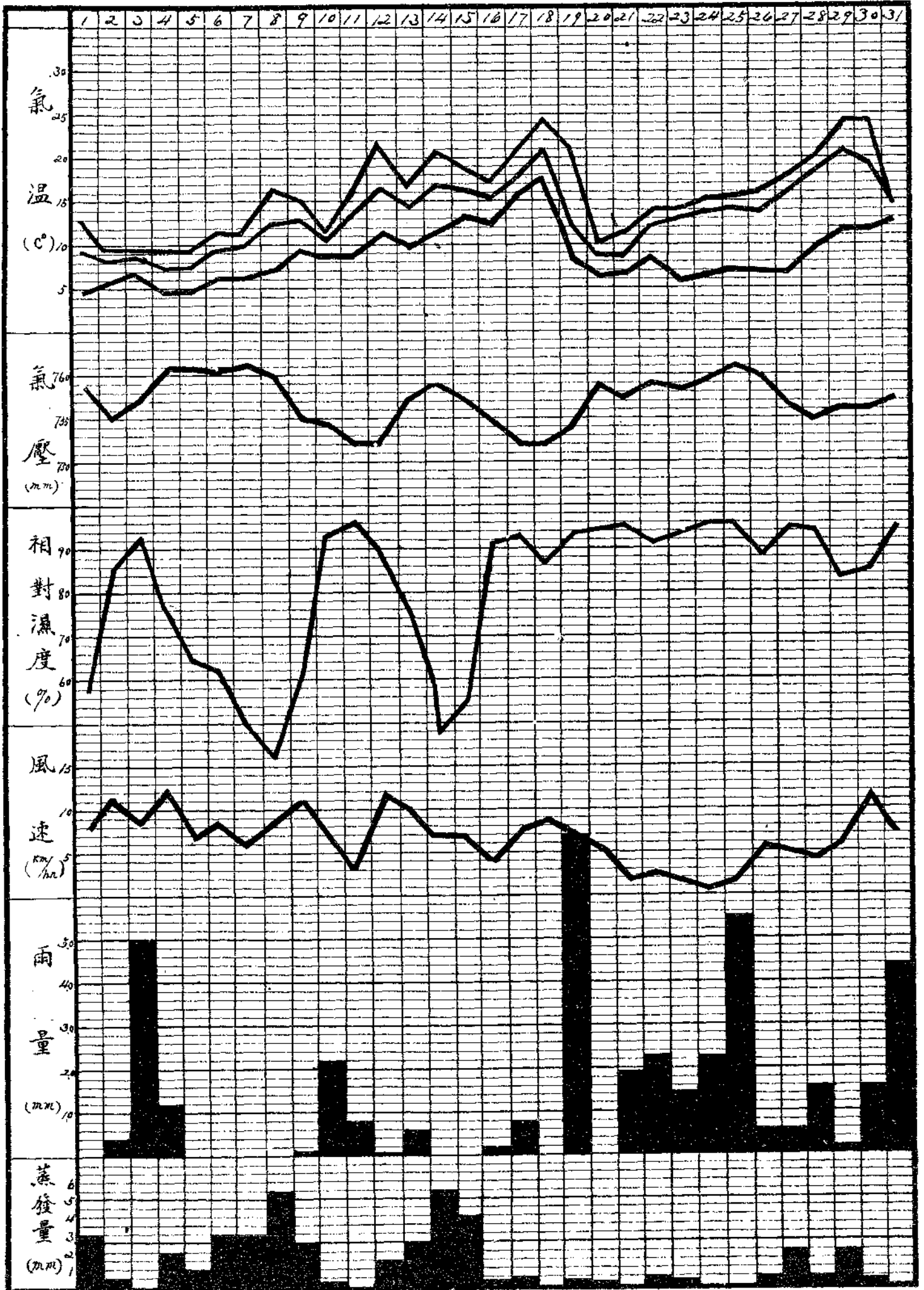
民國二十五年三月份南寧各項氣象要素逐日變遷圖
