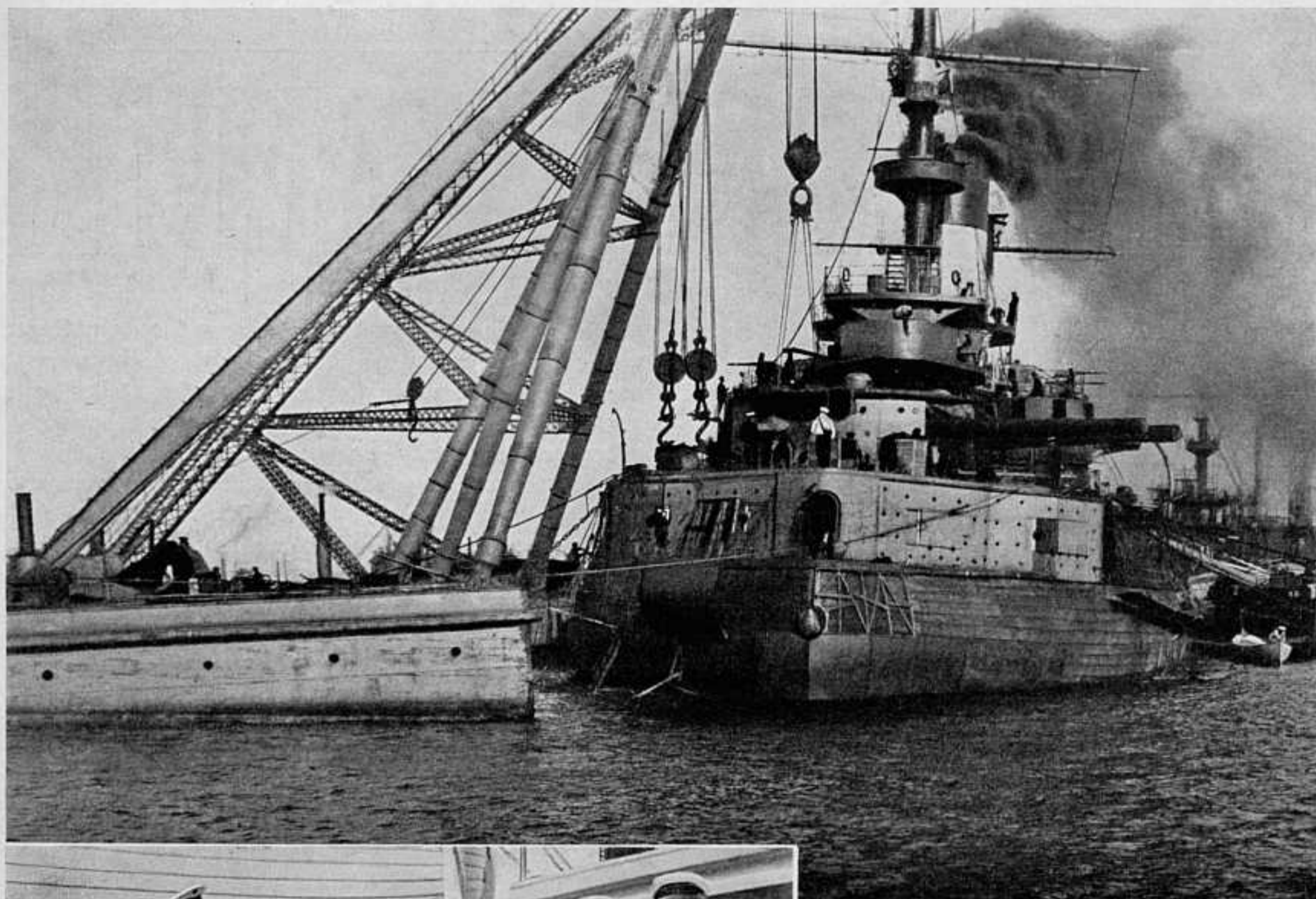
ВООРУЖЕНІЕ ЭСКАДРЕННАГО БРОНЕНОСЦА «СЛАВА». ПОСТАВКА БРОНЕВОЙ ПЛИТЫ.
