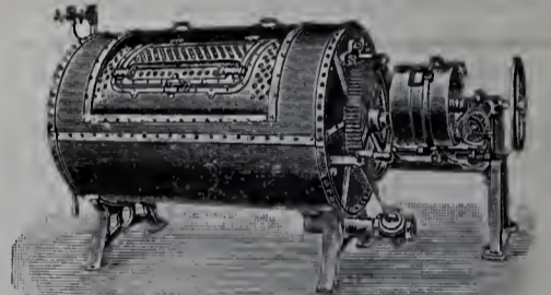
Doppeltrommel-Koch-, Wasch- und Spülmaschine.
