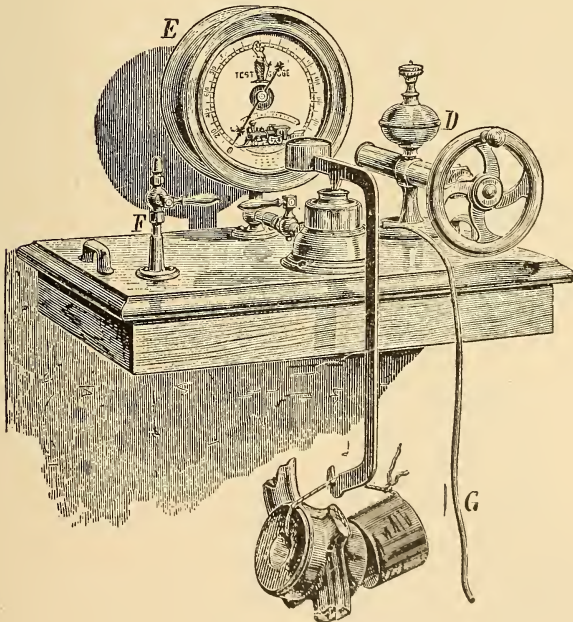
FIG. 41. Utica Gauge Tester.
