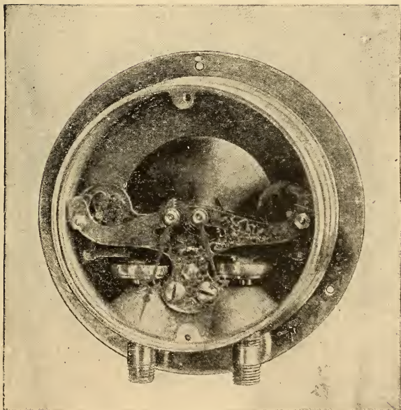
FIG. 32. Utica Duplex Air Gauge.
