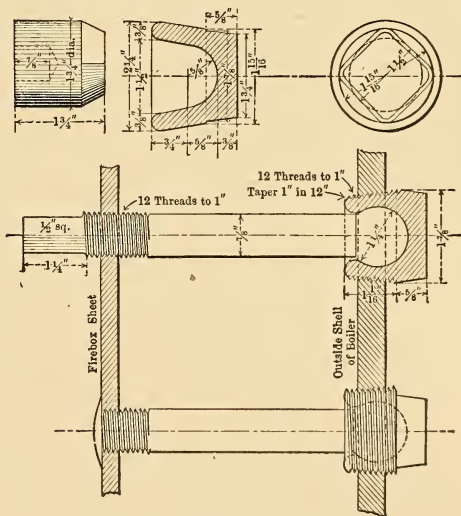
FIG. 1. Johnstone Flexible Stay Bolt.
