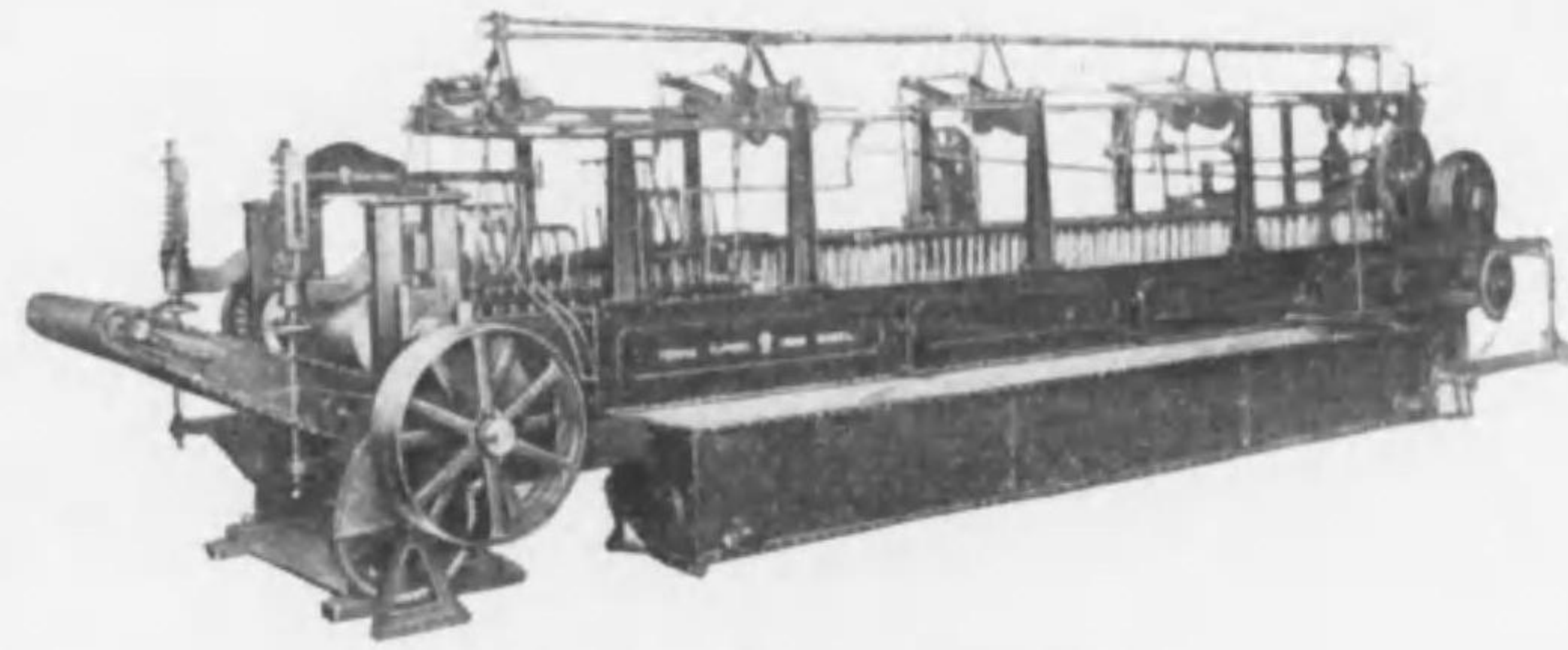
マクノート型洗毛機
