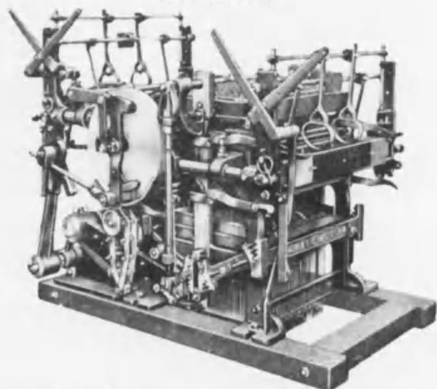
特許 ダブル・シリンダー・クロス・ボーダー ジャカード機
