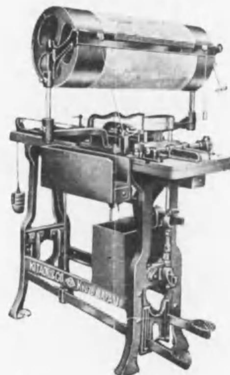
特許ピアノ紋紙穿孔機 (型録御請求次第送呈)
