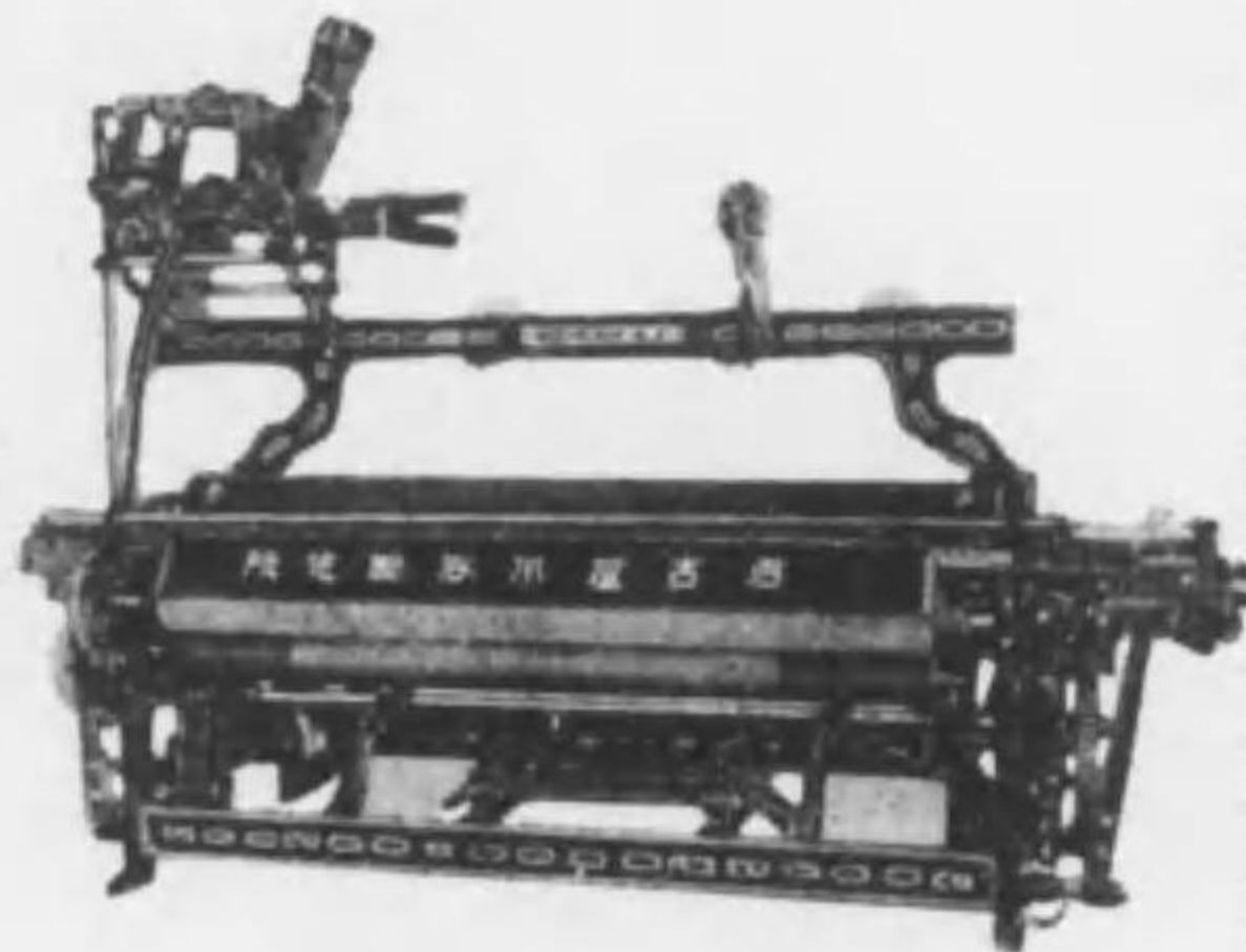
四巾Dビー付織機
