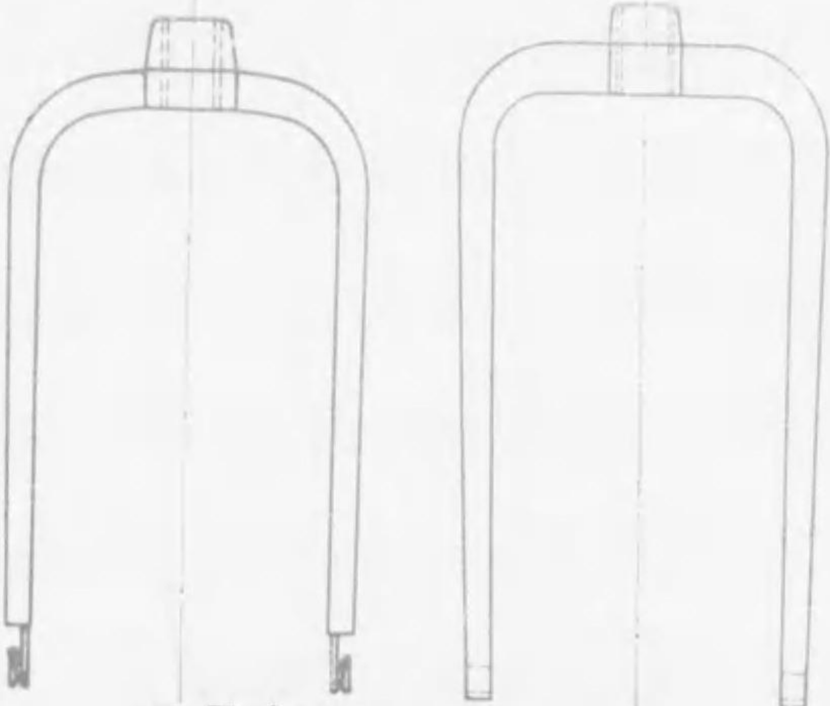
麻紡績用精紡機フライヤー 麻糸用フライヤー
