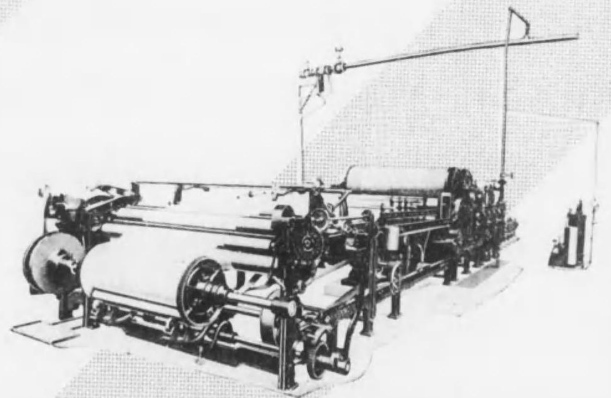
人絹・光棉糸糊附乾燥機
