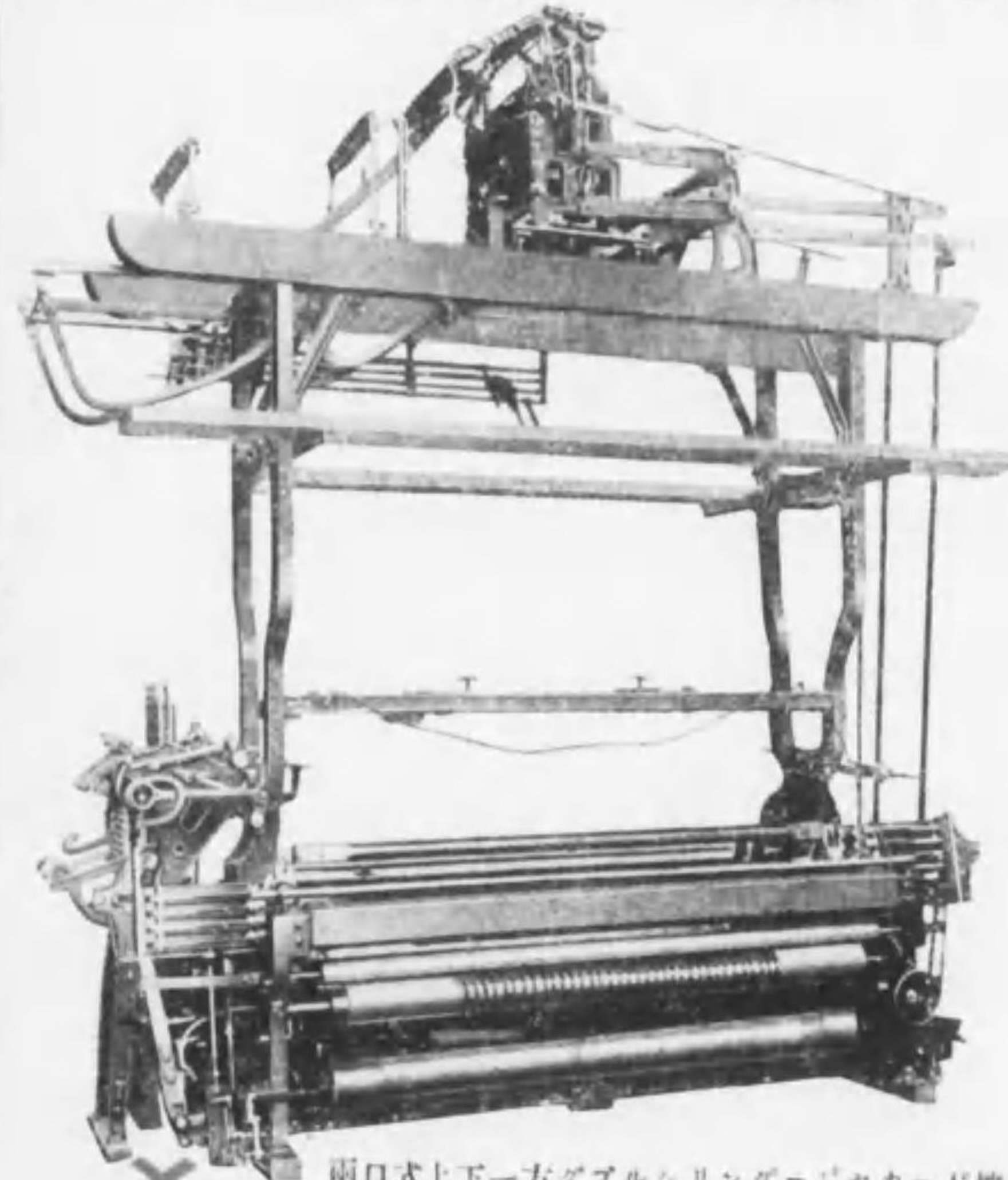
兩口式上下一方ダブルリンドージャカード機
