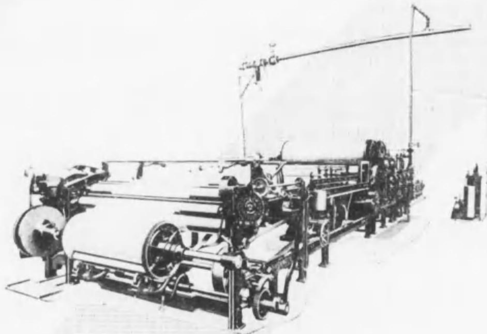
人絹・光棉糸糊附乾燥機
