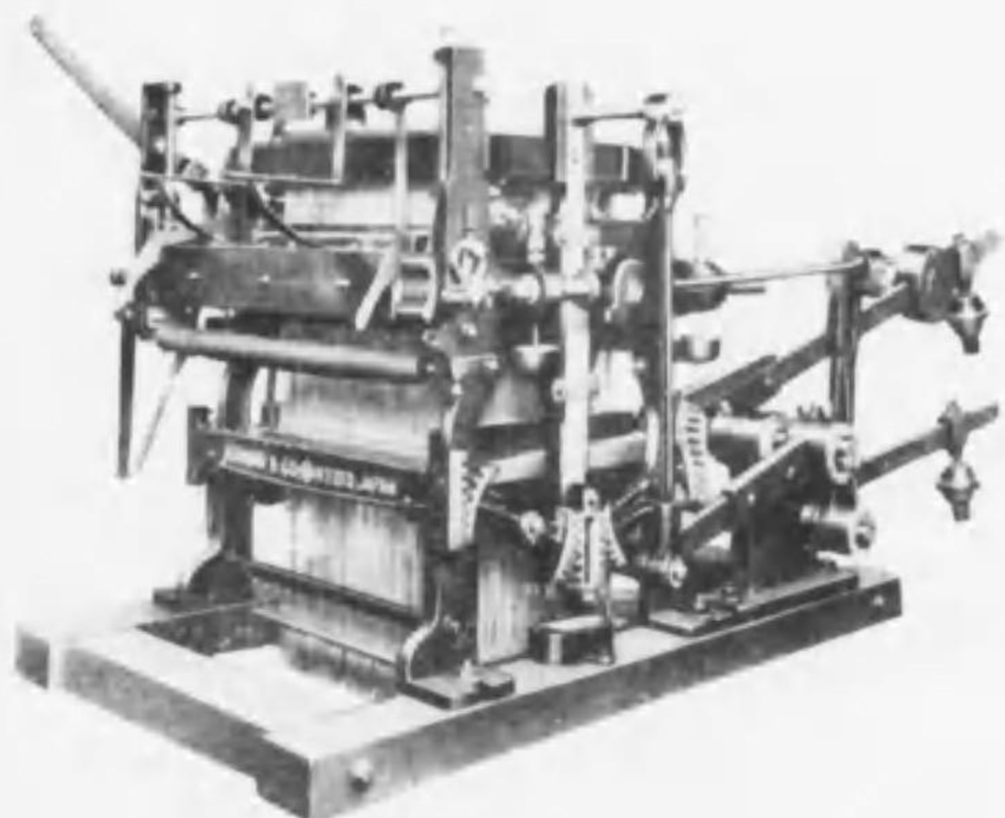
特許兩口式ジャカード機
