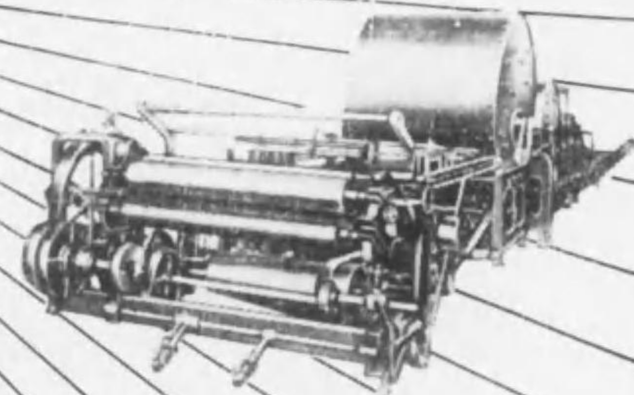
最新型スラツシャー經糸繰付機
