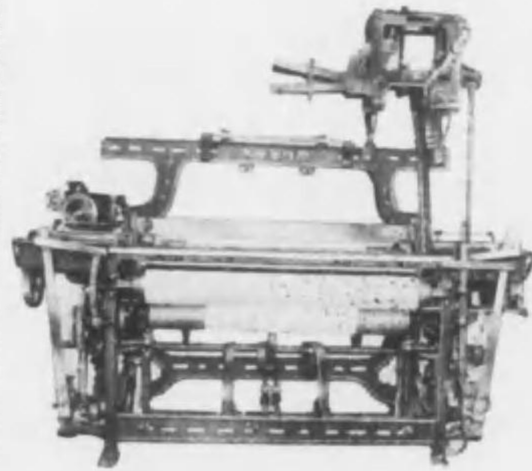
N型兩側二丁杆織機
