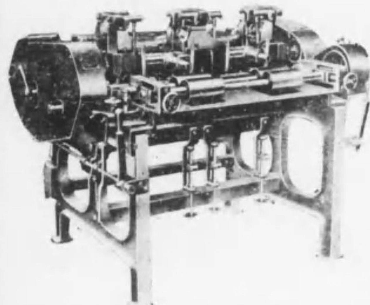
ギル・ボツクス
