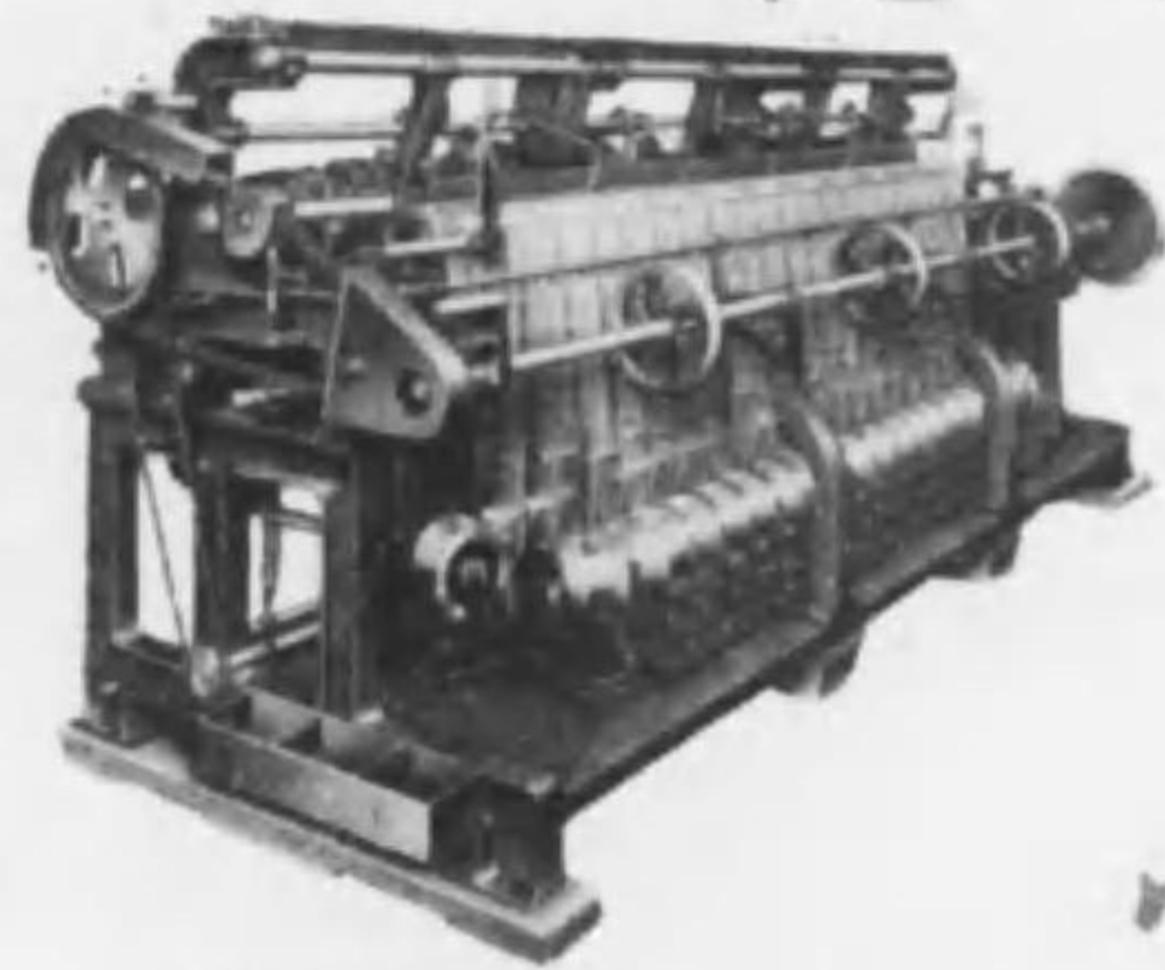
斜交經編機 (ミラノーズ)
