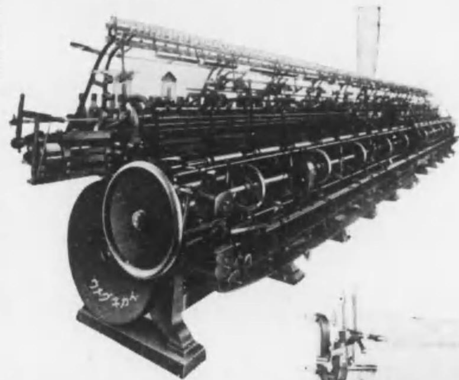
靴下聯成機
