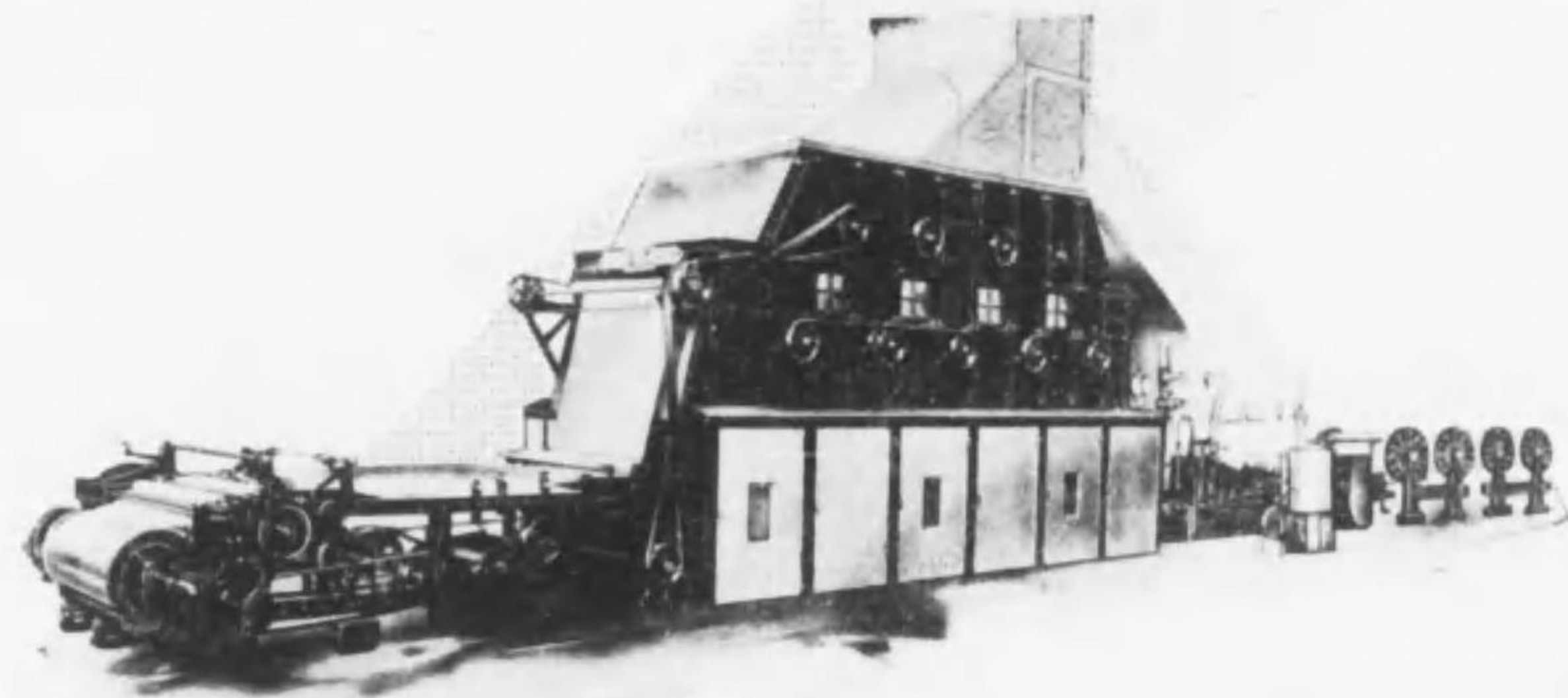
熱風式經糸糊附乾燥機
