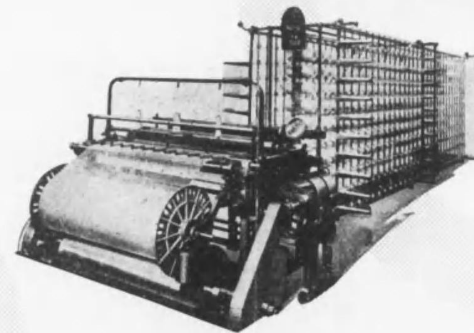
超高速度整經機
