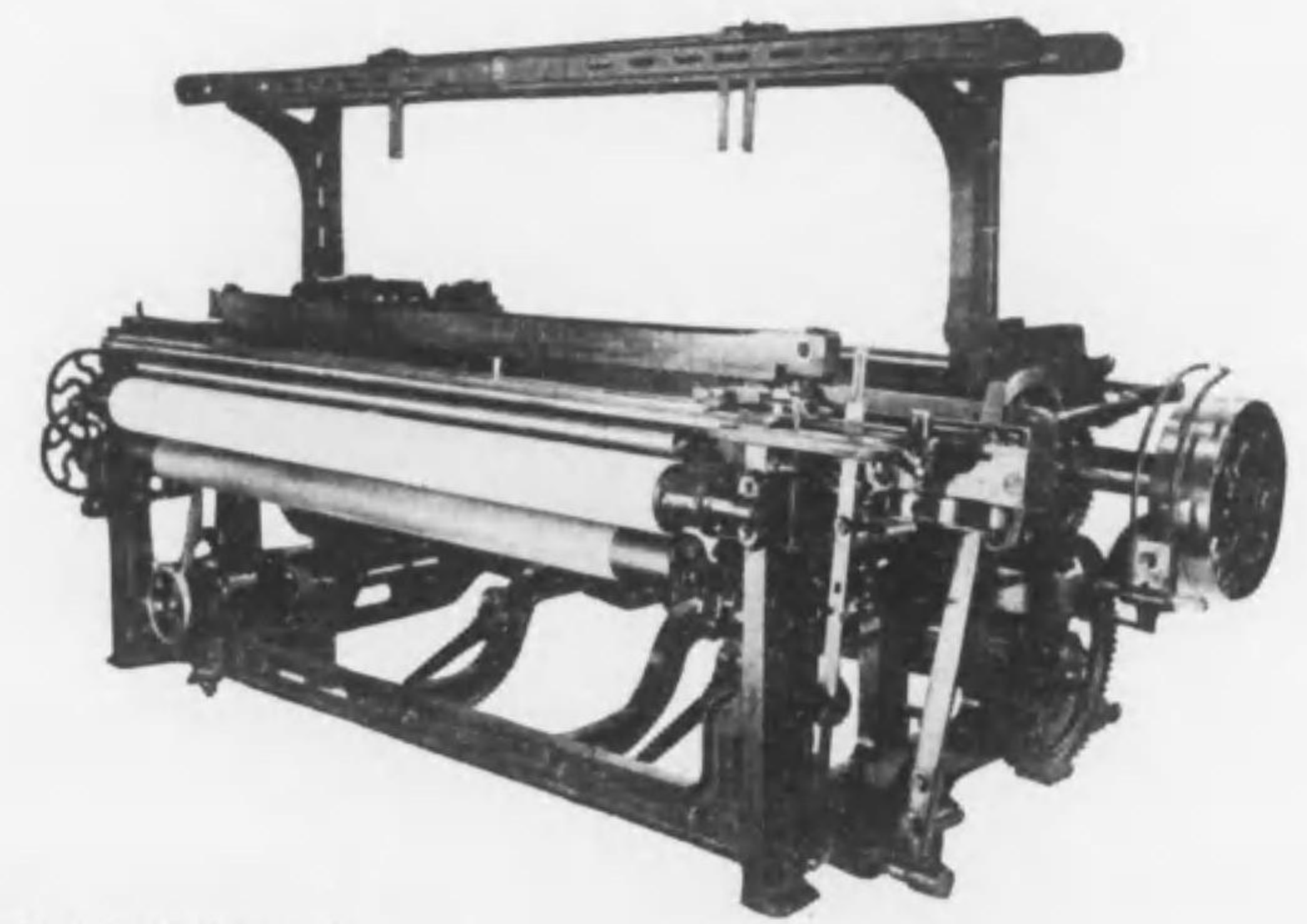
豊田式M型四巾織機
