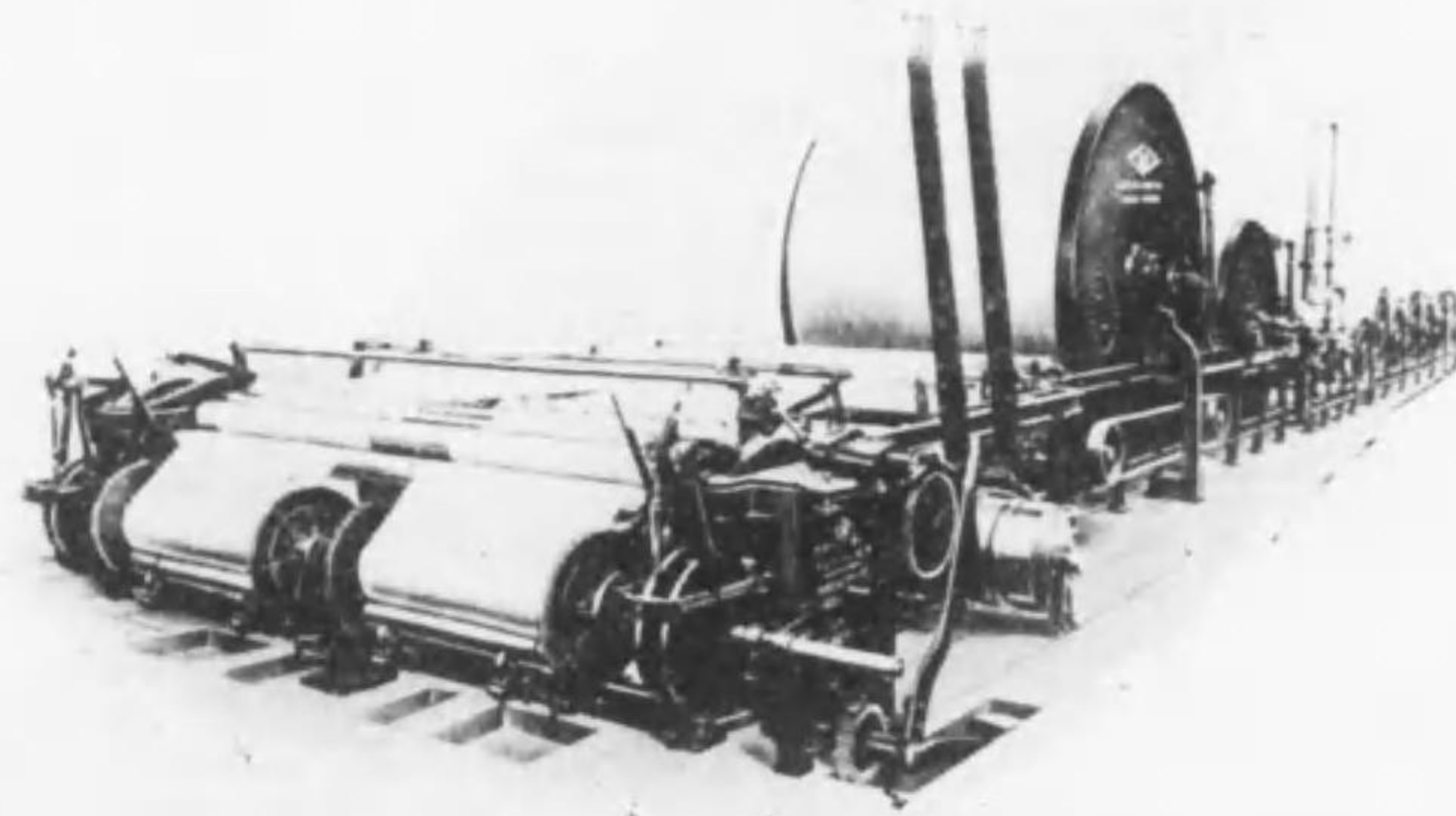
二巾捲取經糸糊附乾燥機
