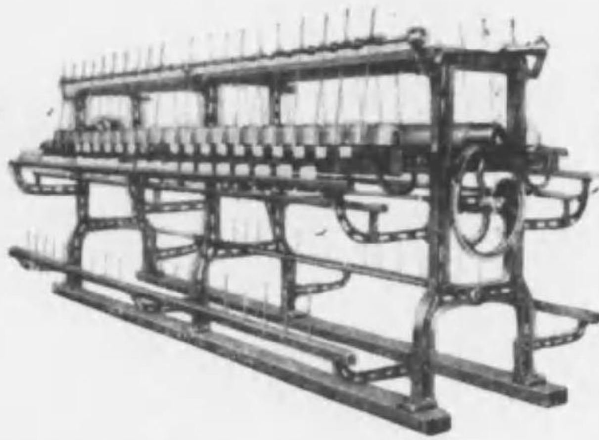
奥井式H型整經機
