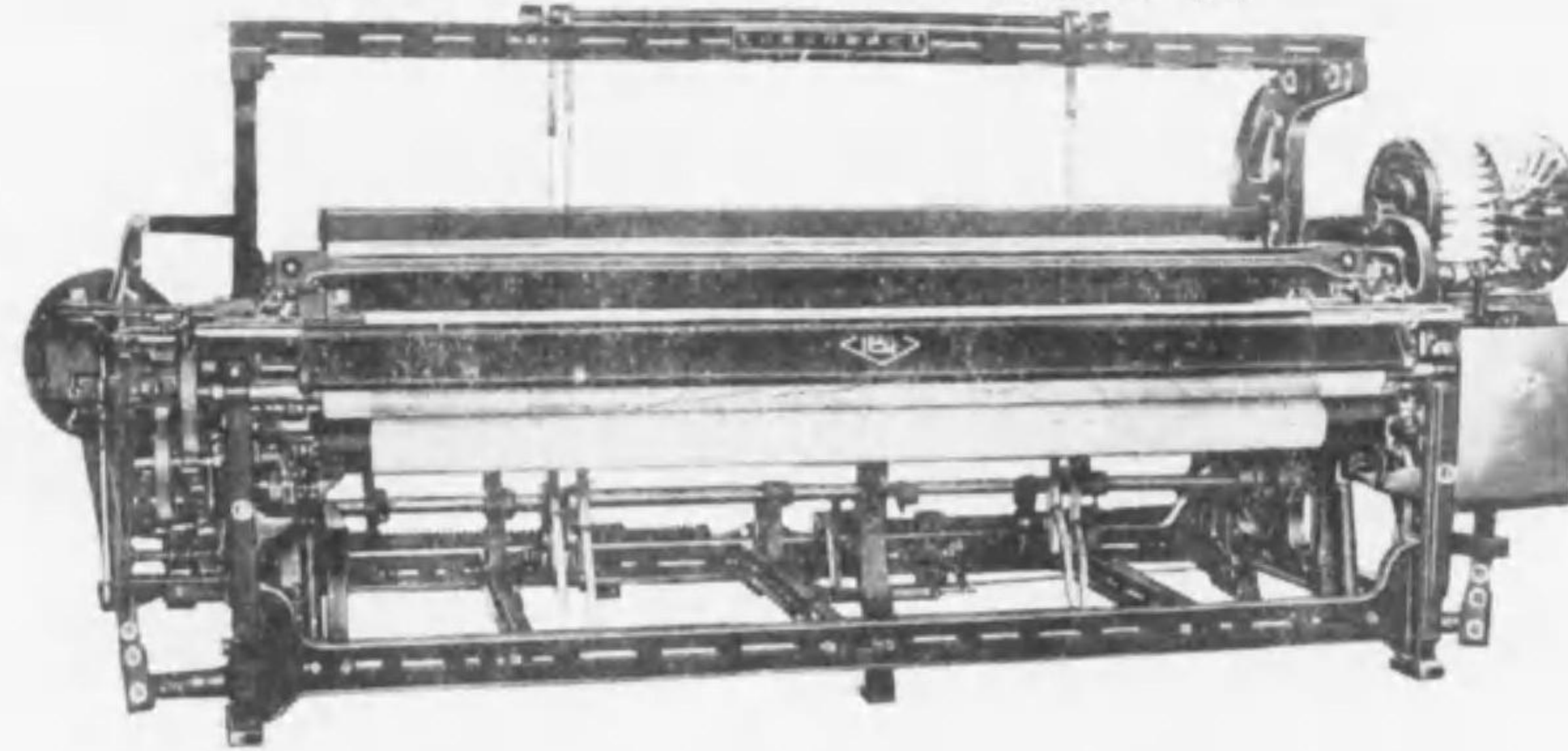
專賣特許 阪本式超廣巾自動織機 箴巾74吋ヨリ120吋迄各種
