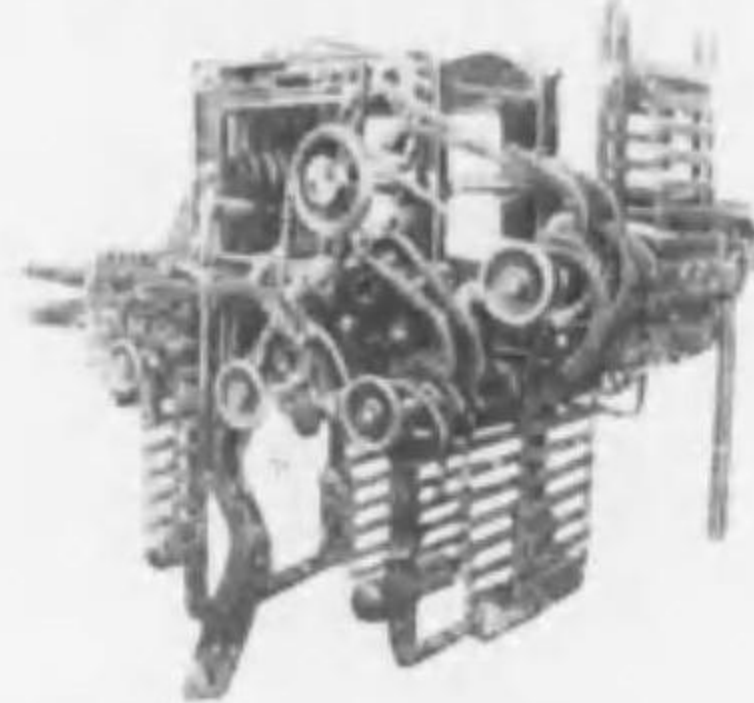
普通ドビー装置
