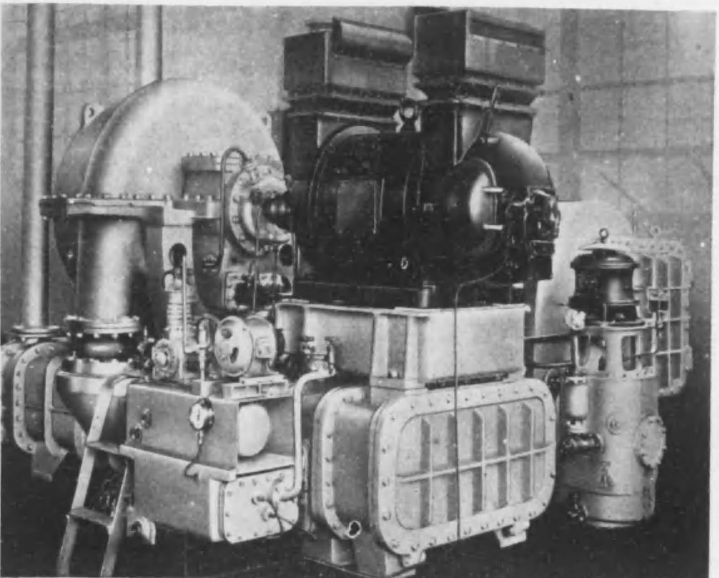
250 噸 420 馬力 ターボ冷凍機
