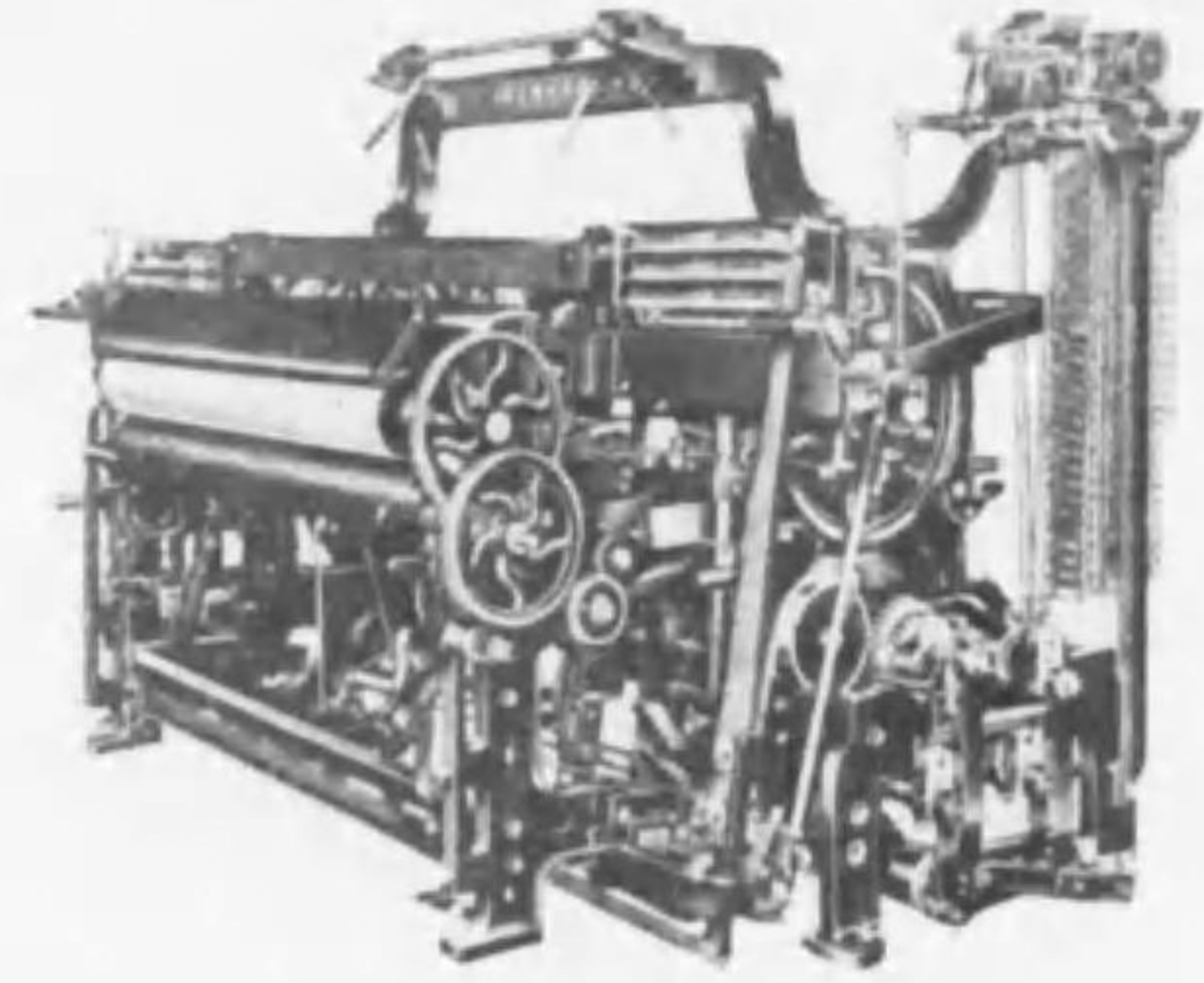
專賣特許 高級織物用 阪本式兩側四挺杼織機
