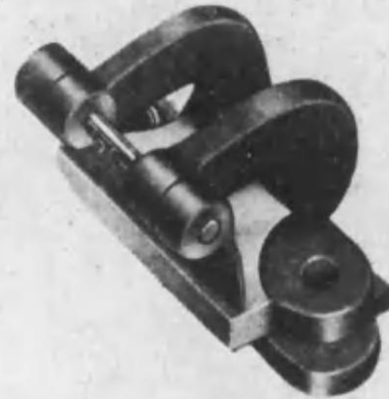
マザー・プラット會社型 シルケツトテンター・クリップ
