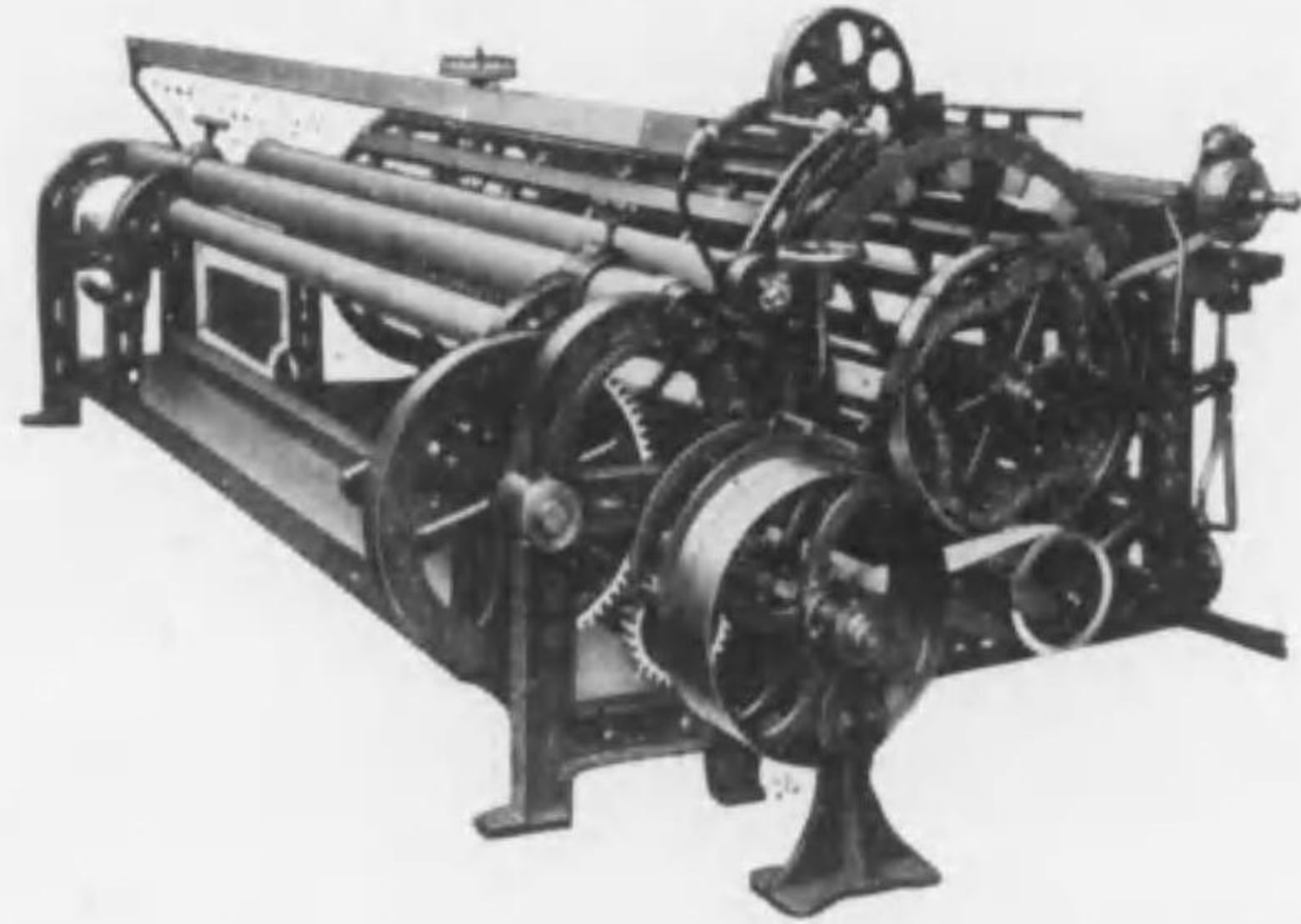
奥井式H型整經機
