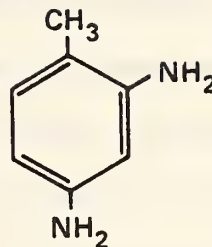
2,4-Diaminotoluene
