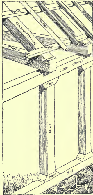
FIG. 7—NEW HAMPSHIRE BARN FRAME
