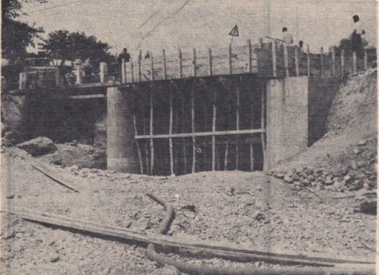
علیات بتون ریزی بل سیاه رود شاهی
