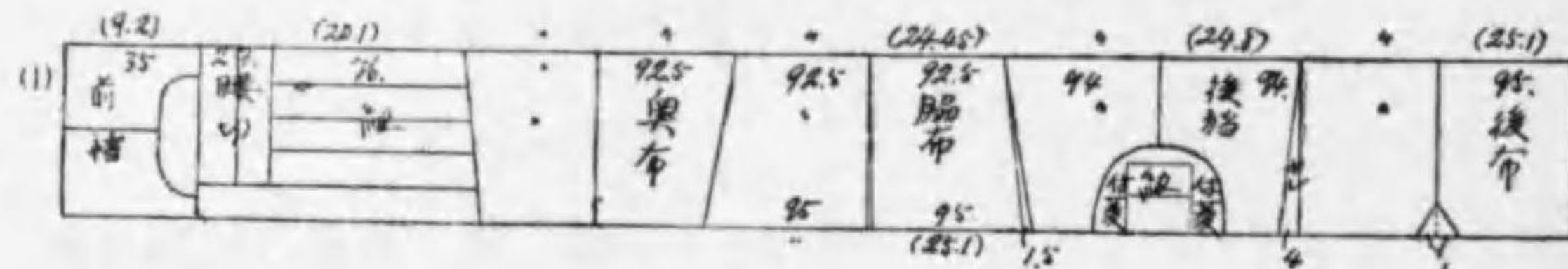
◎並幅の布を以て男物拾番馬乗袴の裁方及び積り方
