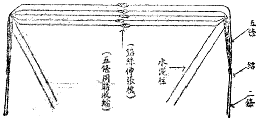
狀之緊收部中棚在絲鉛 圖四五第
