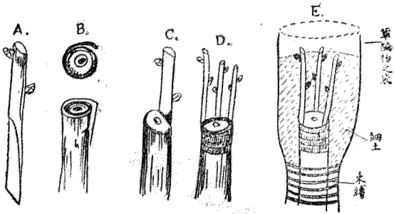
(接高)接袋 圖四三第
