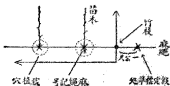
況狀之準標繩麻時栽植 圖三四第 (圖面平)
