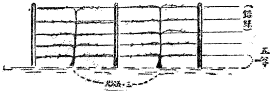
形骨肋平水 圖九六第
