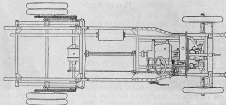
Видъ сверху.
