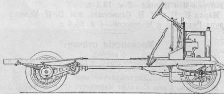
Видъ сбоку.
