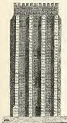
Fig. 264. Donjon.
