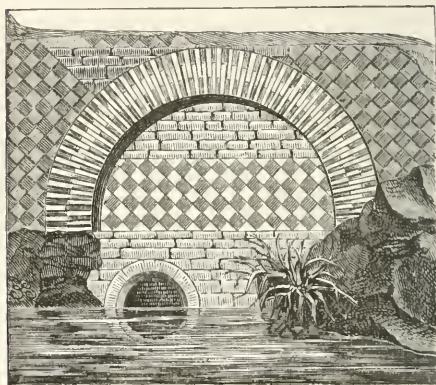
Fig. 583. Reticulatum opus.
