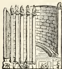
Fig. 560. Præfurnium hypocaust.
