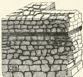
Fig. 504. Pseudisodorum opus, with a course of opus insertum.
