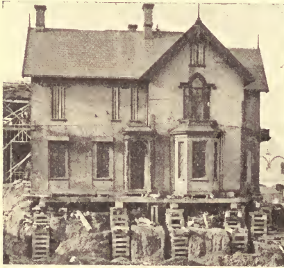
Aspect d'une maison en cours de déplacement.
