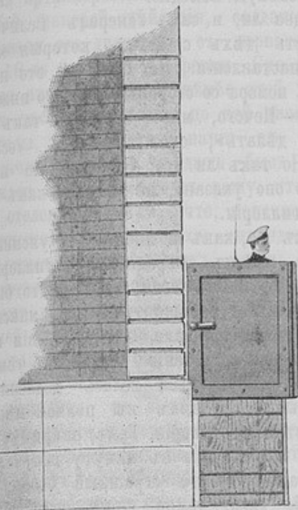
Черт. № 2. Видъ сбоку.
