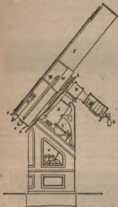
Фиг. 5. Установка рефлектора Кассегрена. A — полярная ось, B — ось склоненій, и — часовой механизмъ, F — рефлекторъ, о — окуляръ, S — искатель.
