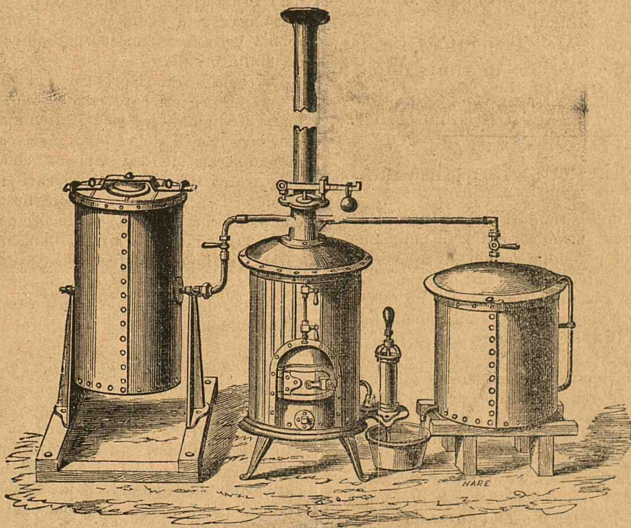
Aparate de copt cu abur (a se vedea articolul relativ din acest număr.
