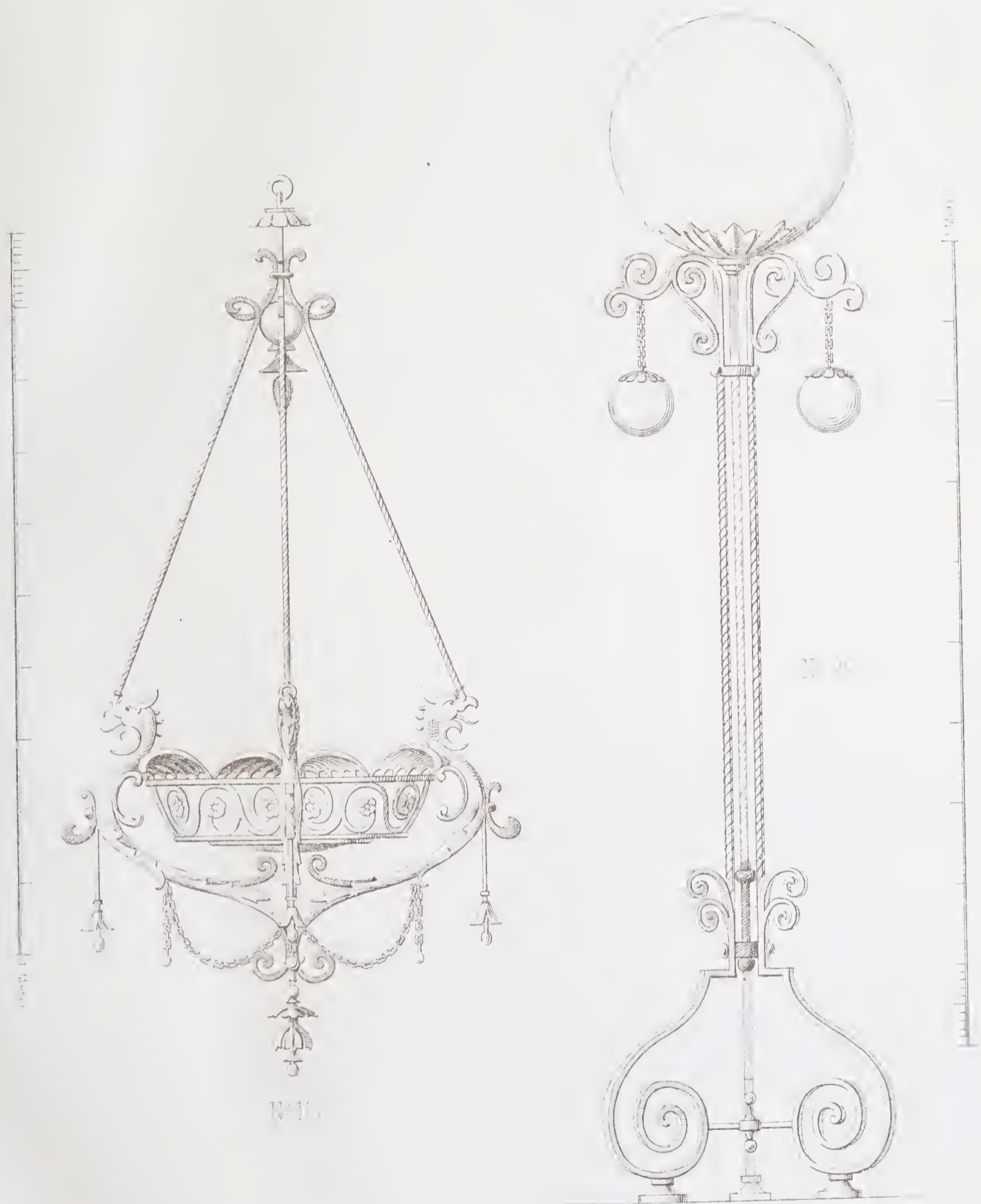
Blumenkugel und Gartenlampe mit Glaskugeln Eisen und Messing in der Bauhütte und Fabrik schmiedeeisener Ornamente von F. PULS in Berlin, Holzmarkt-Str. 13.
