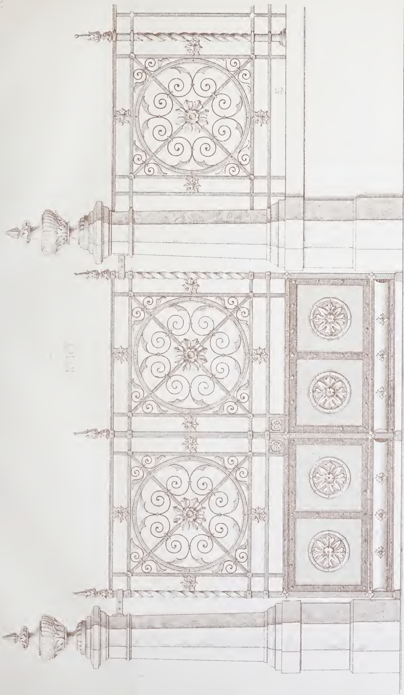
Thürweg u. Gitter zum Hause des Gehrnigen Commerzienrathes Wihl Conrad in Berlin.
