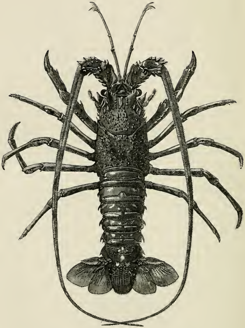
FIG. 70. Palinurus vulgaris (about \frac{1}{4} nat. size).
