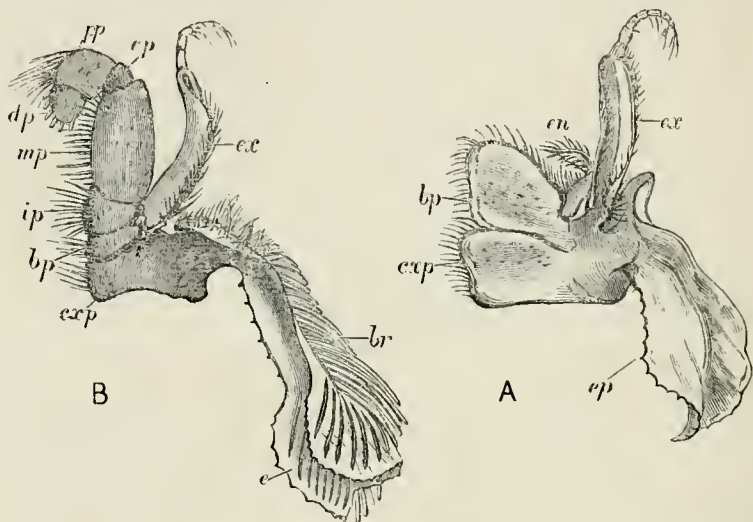
FIG. 45.— Astacus fluvialtilis .—A, the first; B, the second maxillipede of the left side ( \times 3 ). exp , coxopodite; bp , basipodite; c, br , podobranchia; ep , epipodite; en , endopodite; ex , exopodite; ip , ischiopodite; mp , meropodite; cp , carpopodite; pp , propodite; dp , dactylopodite.
