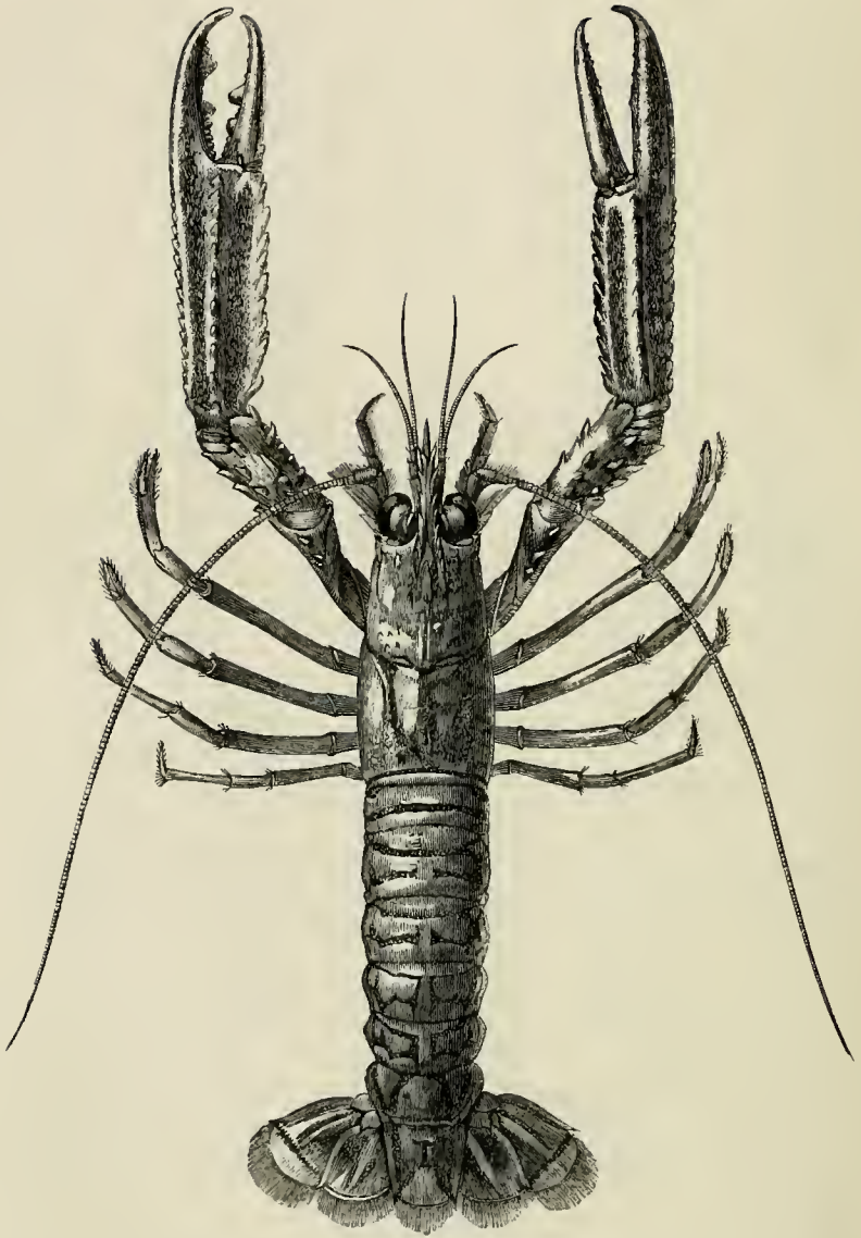
Fig. 69. Nephrops norvegicus ( \frac{1}{2} nat. size).
