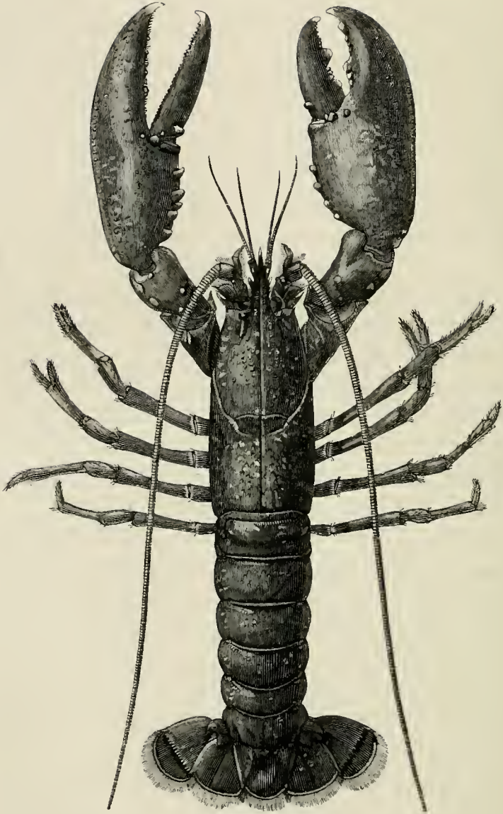
FIG. 67. Homarus vulgaris ( \frac{1}{3} nat. size).
