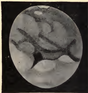
Fig. 52.—Drawing of Mars (August 16th, 1894).
