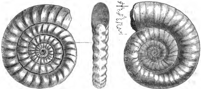
Pylon. laevis.
