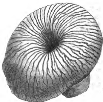
Cnemidium Goldfussii.
