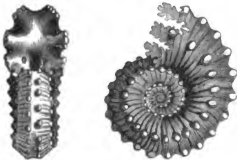
Ammonites ornatus.
