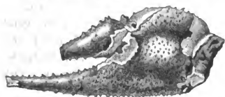
Glyphaea Aalensis .
