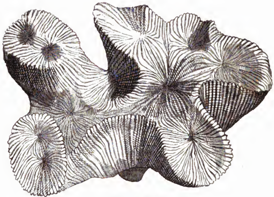
Lobophyllia suevica.
