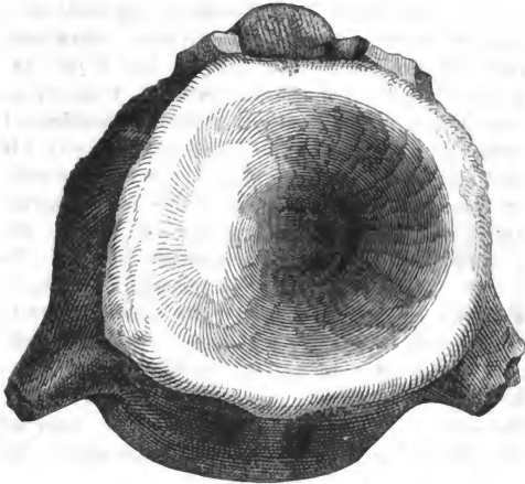
Termatosaurus. Plesiosaurus?
