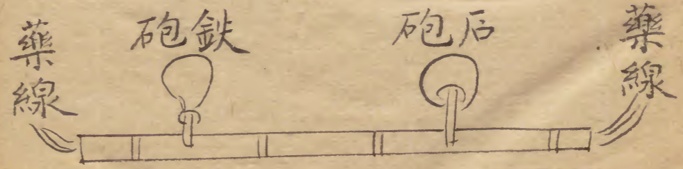
地坑埋伏石砲生鉄砲引薬線竹式
