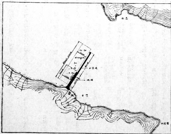
隴海鐵路連雲港老窰碼頭建築計畫略圖
