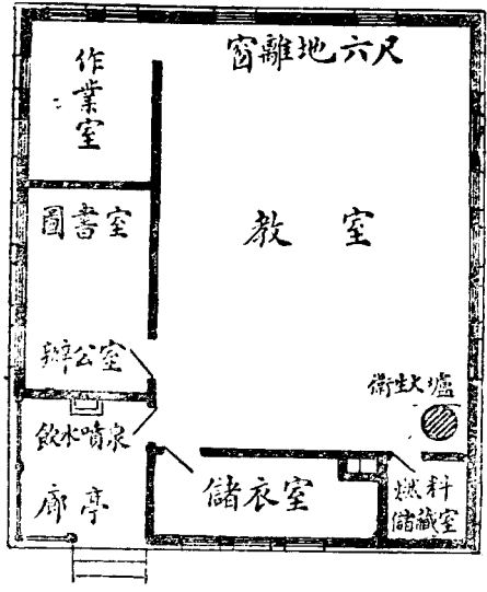
最經濟的單級鄉村學校平面圖
