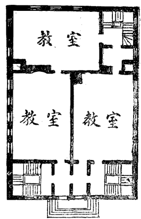
阿拉白馬學校底層之平面圖
