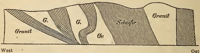
Grenze zwischen Granit und Schiefer bei S. Piero.
