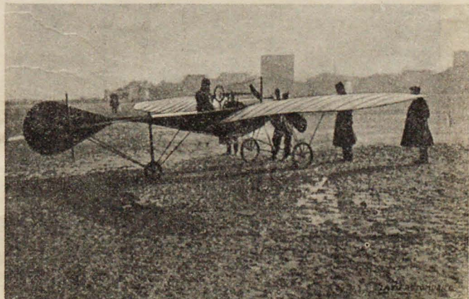
Монопланъ Муассана; поддерживающая поверхность 12 кв. м.; моторъ Гномъ въ 50 лощ. с.
