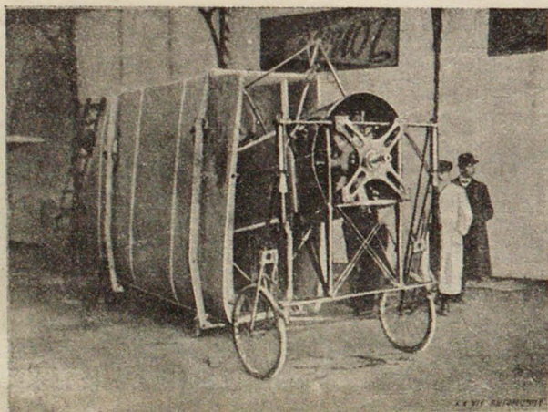
Монопланъ Жака Бальзана, упакованный для отправки въ Египетъ.]
