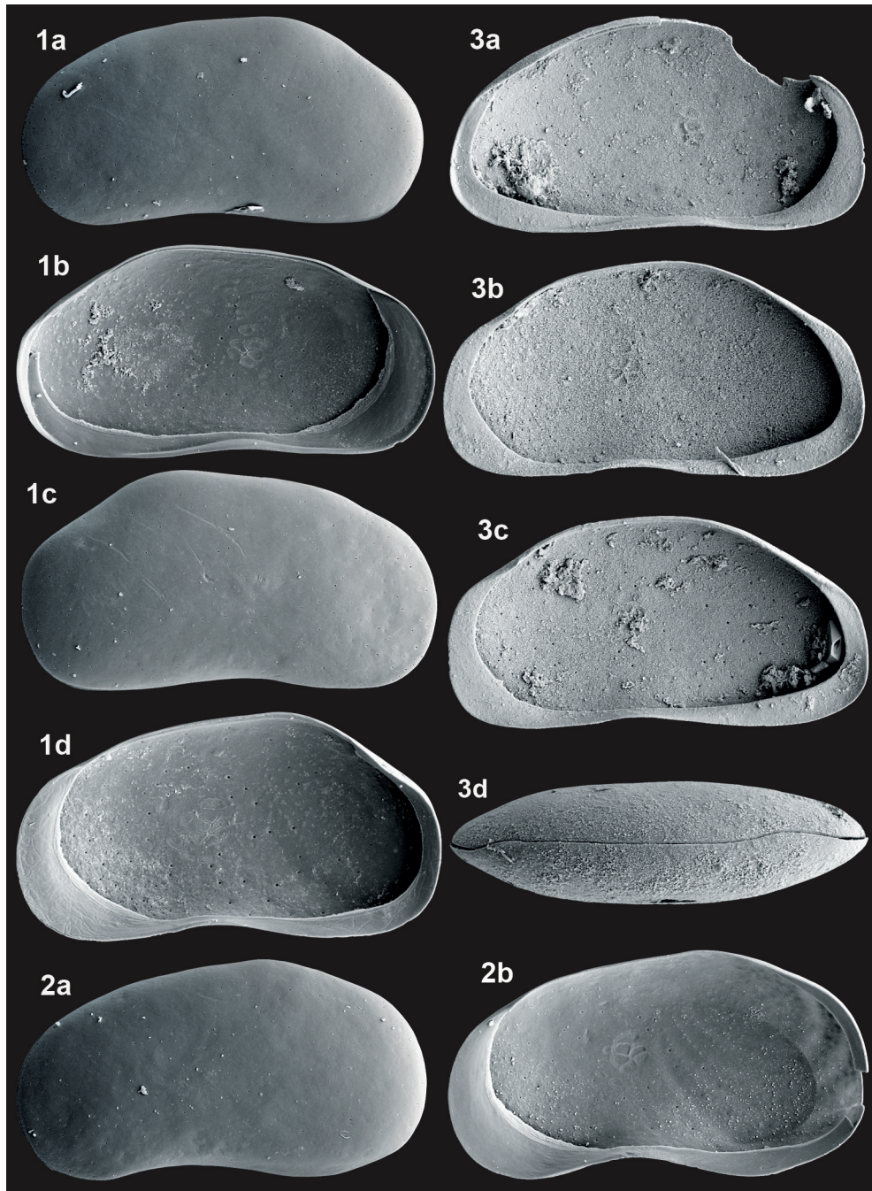
Fabaeformiscandona fabella (NÜCHTERLEIN, 1969) – Svaty Ondrej (SK) Ho Weibchen: 1a - LVa (L 0,55), 1b - LVi (L 0,61), 1c - RVa (L 0,53), 1d - RVi (L 0,57), Männchen: 2a - LVa (L 0,60), 2b - RVi (L 0,60).
