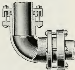
Fig. 96—90 DEG. ELL
