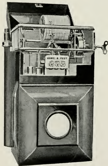
Fig. 201—COMPLAINT METER
