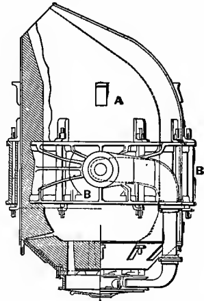
FIG. 54.—CONVERTER.
