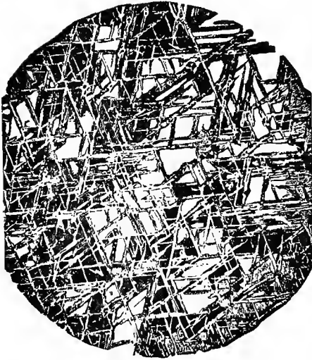
FIG. 124.—METEORIC IRON.
