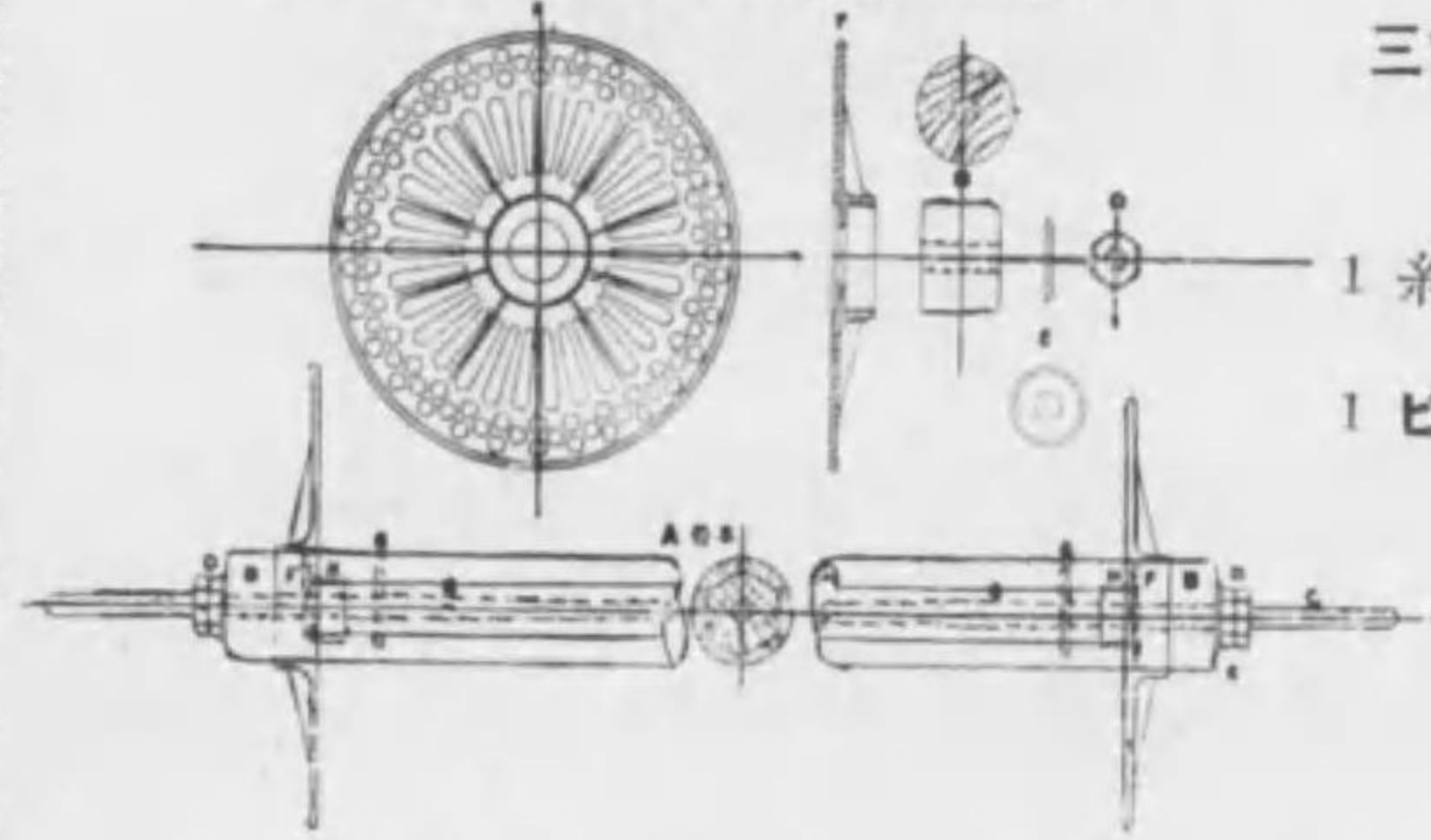
三ツワ式特製新型荒卷ビーム
