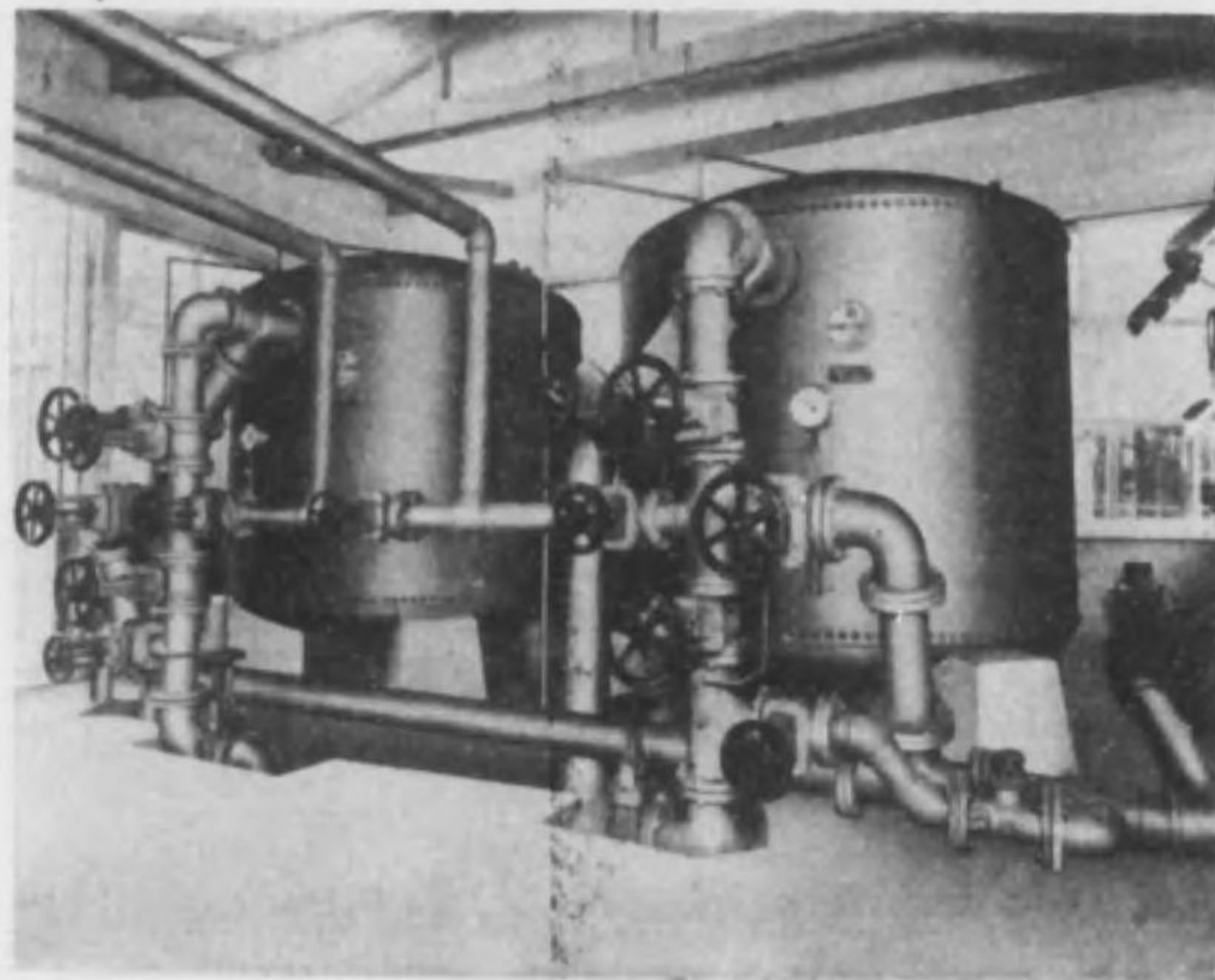
急速濾水裝置
