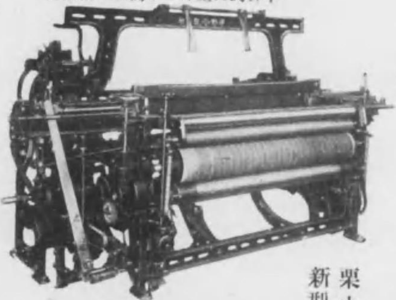
平野式H型二片高丁綴人絹織機
