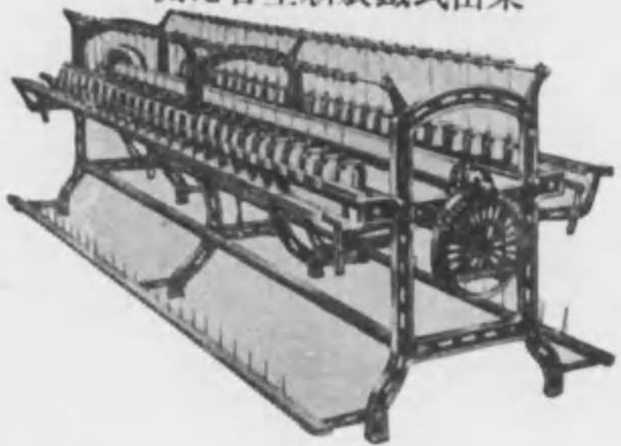
栗山式新製鐵管捲機
