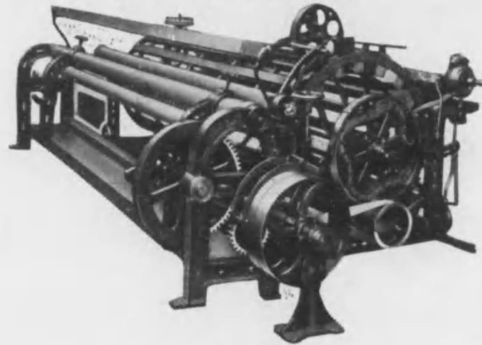
奧井式H型整經機
