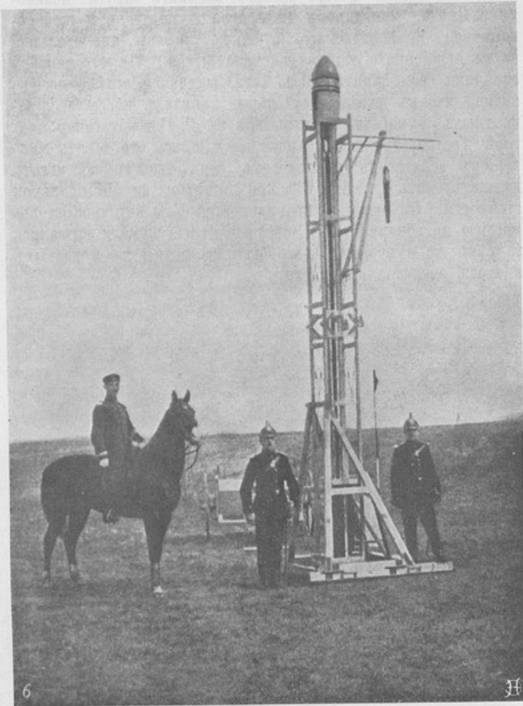
Ракета Мауля для производства фотографических снимков местности, испытываемая в Германіи.
