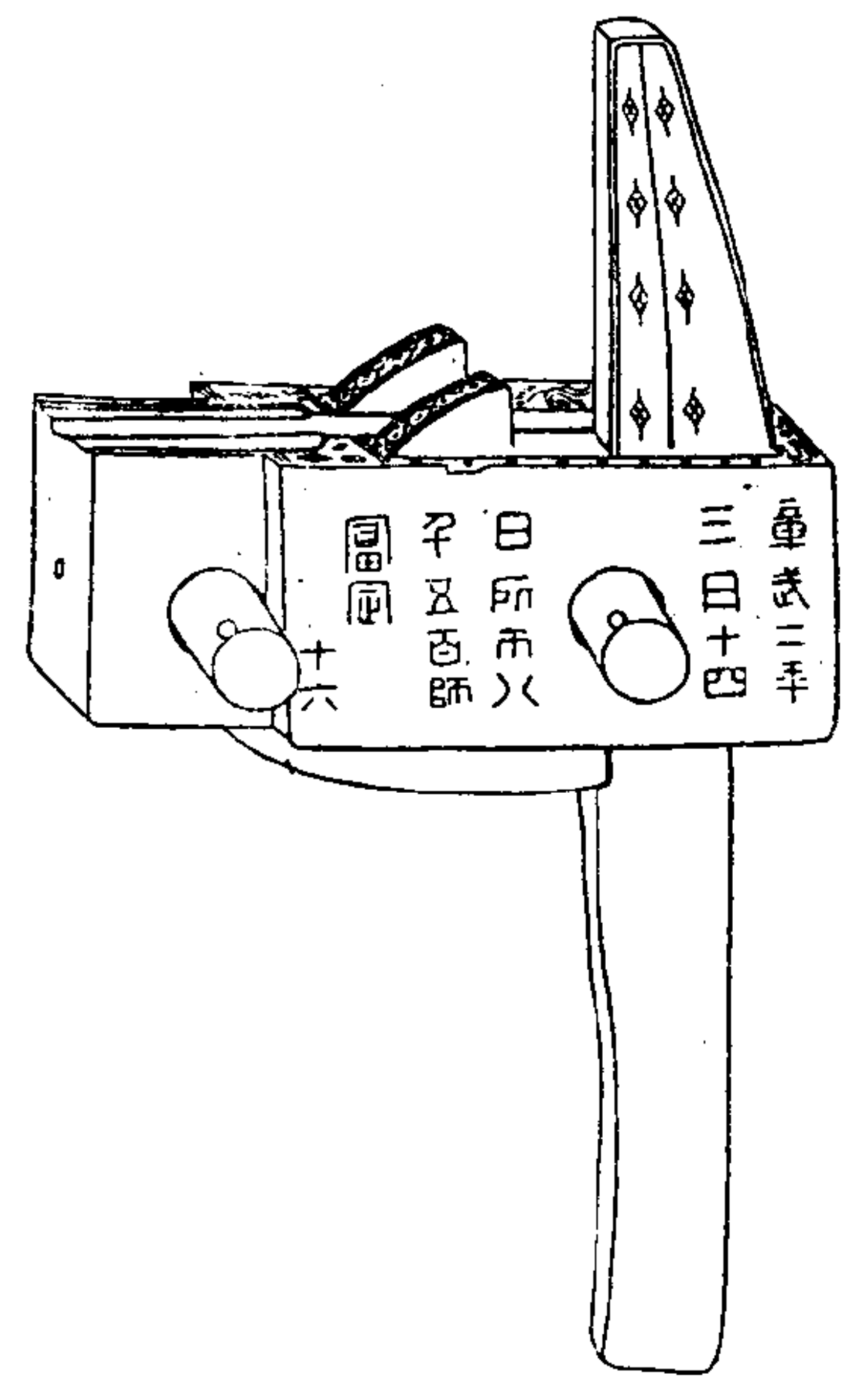
蜀漢章武弩機 原形
