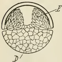
Fig. 5. Lithionembryo.
